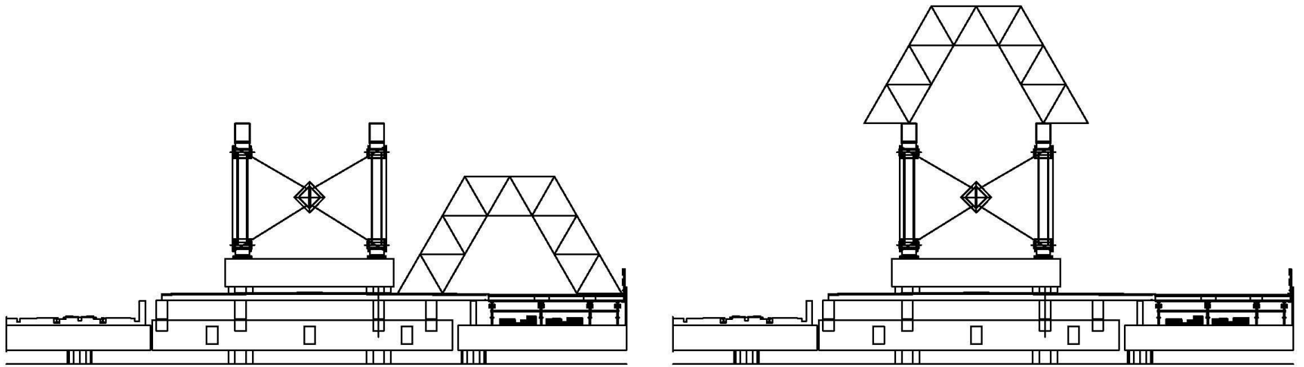
Figuur 1: Vooraf opbouwen van centraal in kap gelegen ruimtevakwerk secties op perronniveau + in hijsen.
