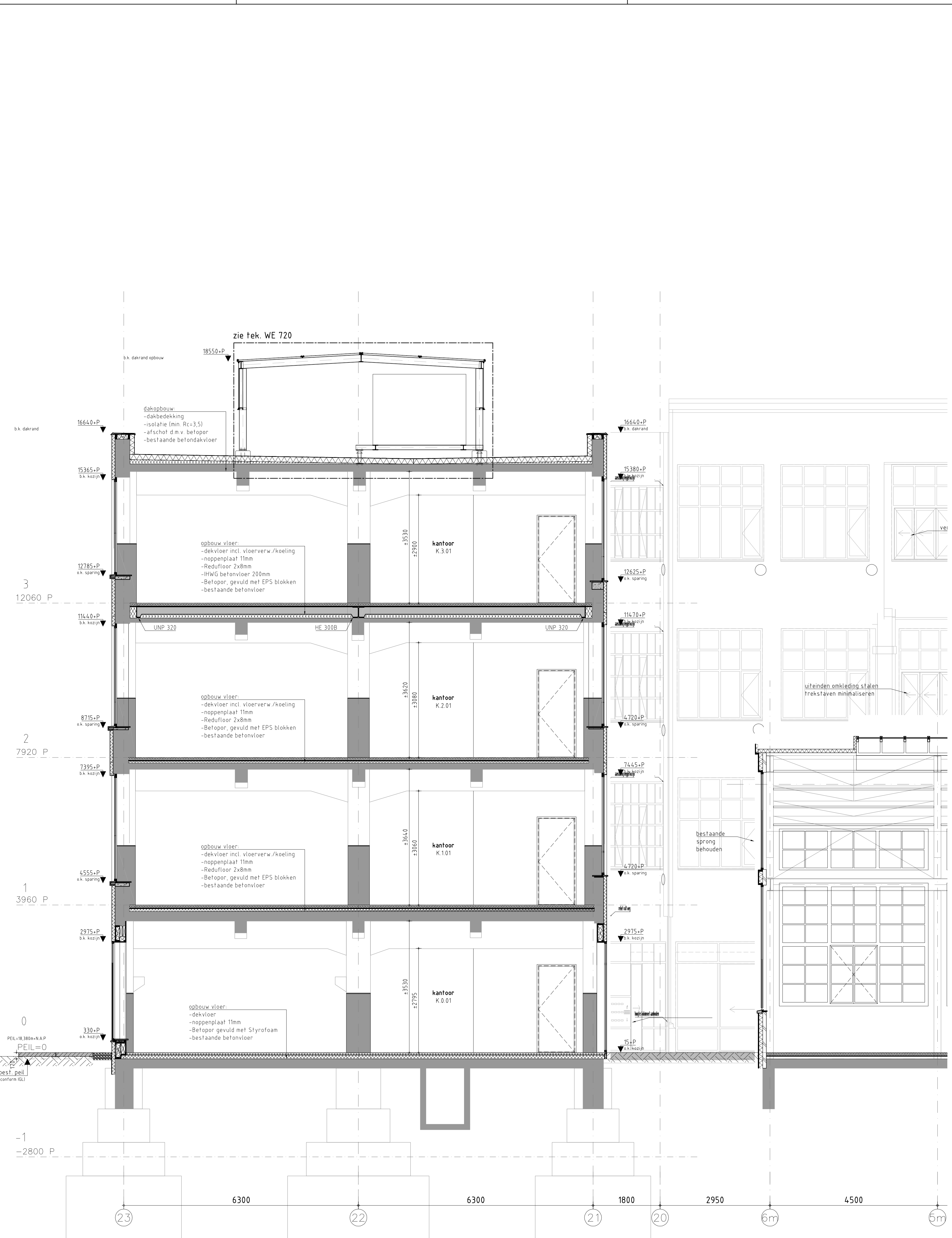
doorsnede 2
