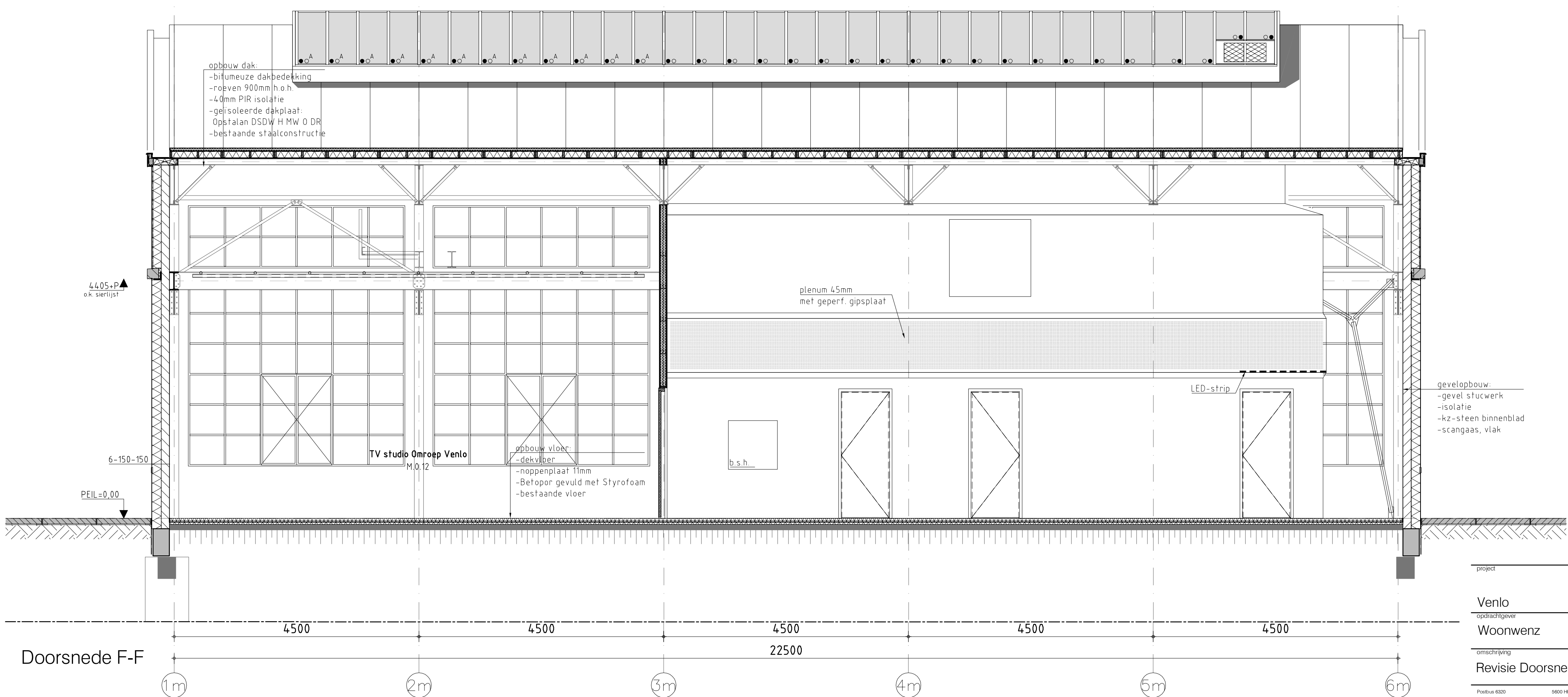
Doorsnede D-D
