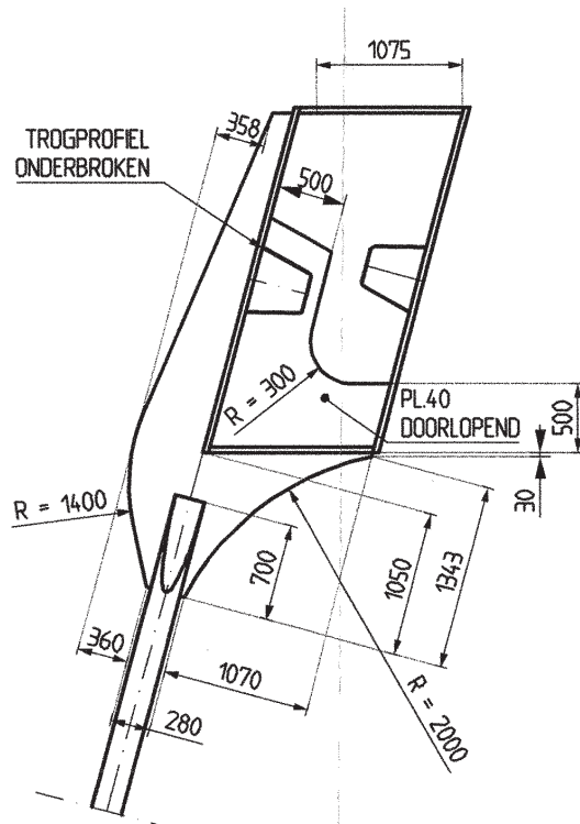
PRINCIPE DETAIL HANGER 3 EN 4
