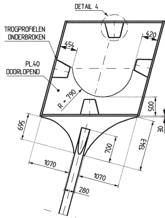
PRINCIPE DETAIL HANGER 1 EN 2
