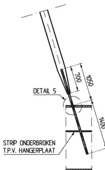
PRINCIPE DETAIL HANGER 1 EN 2
