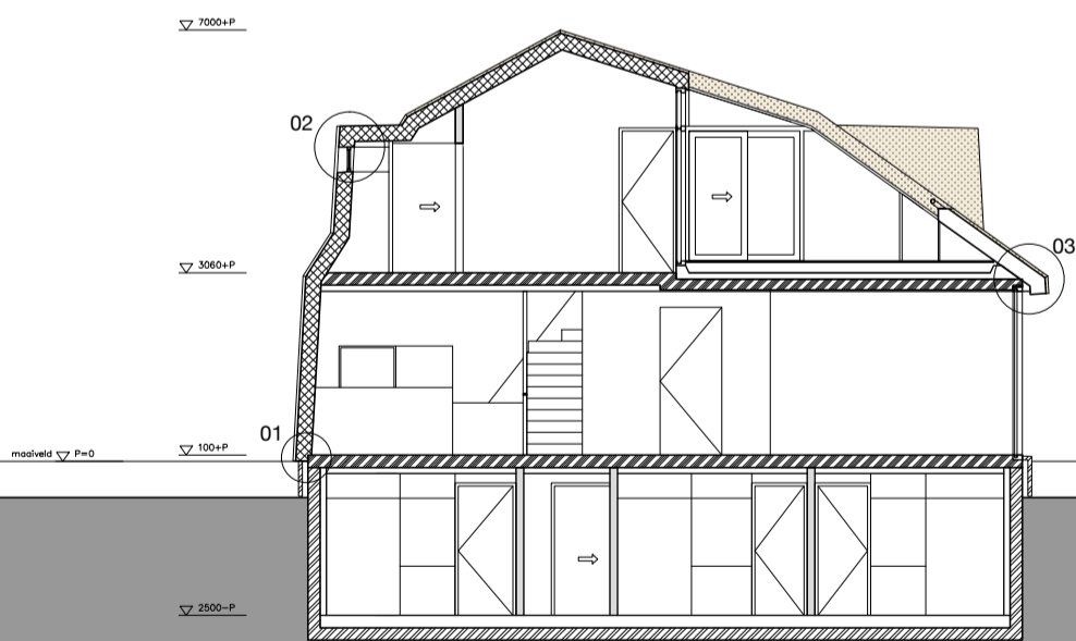
langsdoorsnede A
