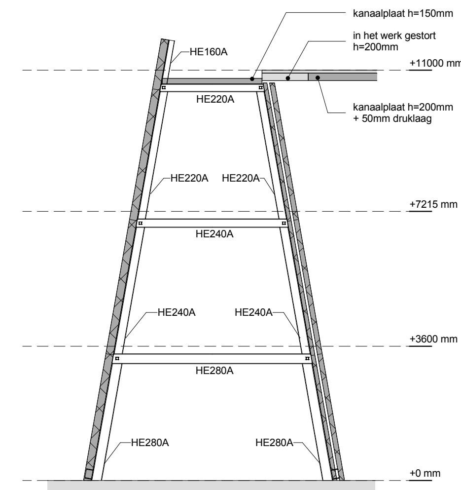
Doorsnede H-H
