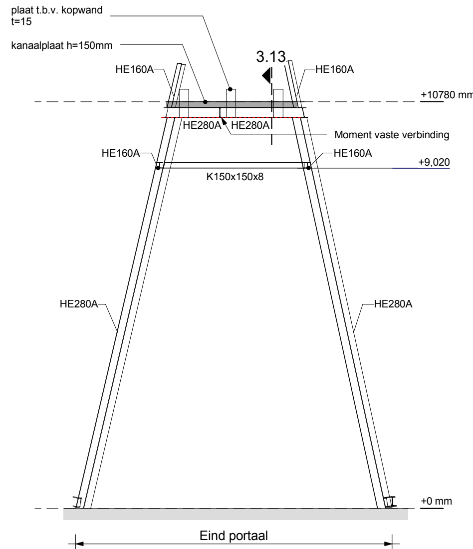
Doorsnede I-I
