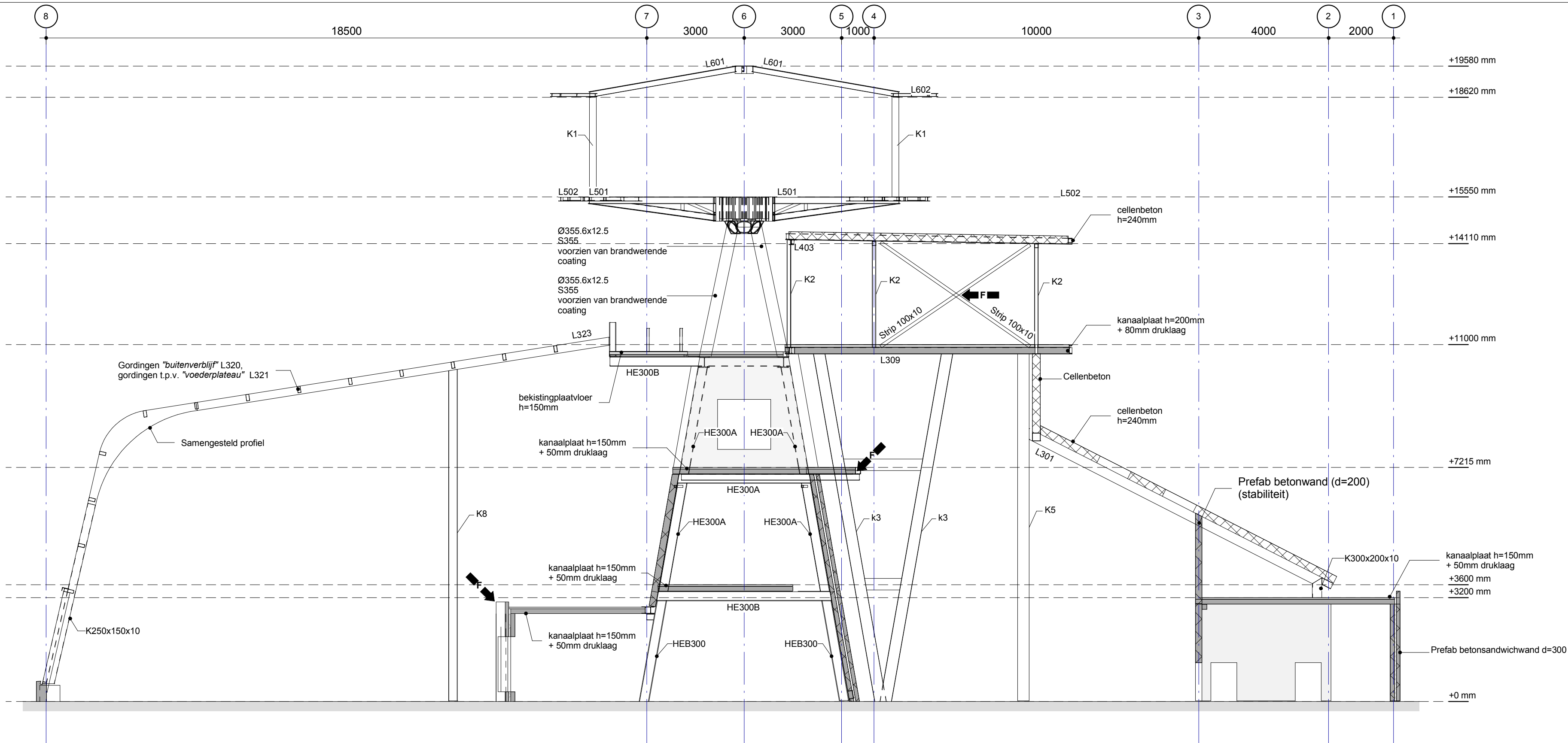
Doorsnede F-F
