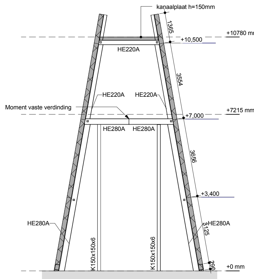
Doorsnede J-J
