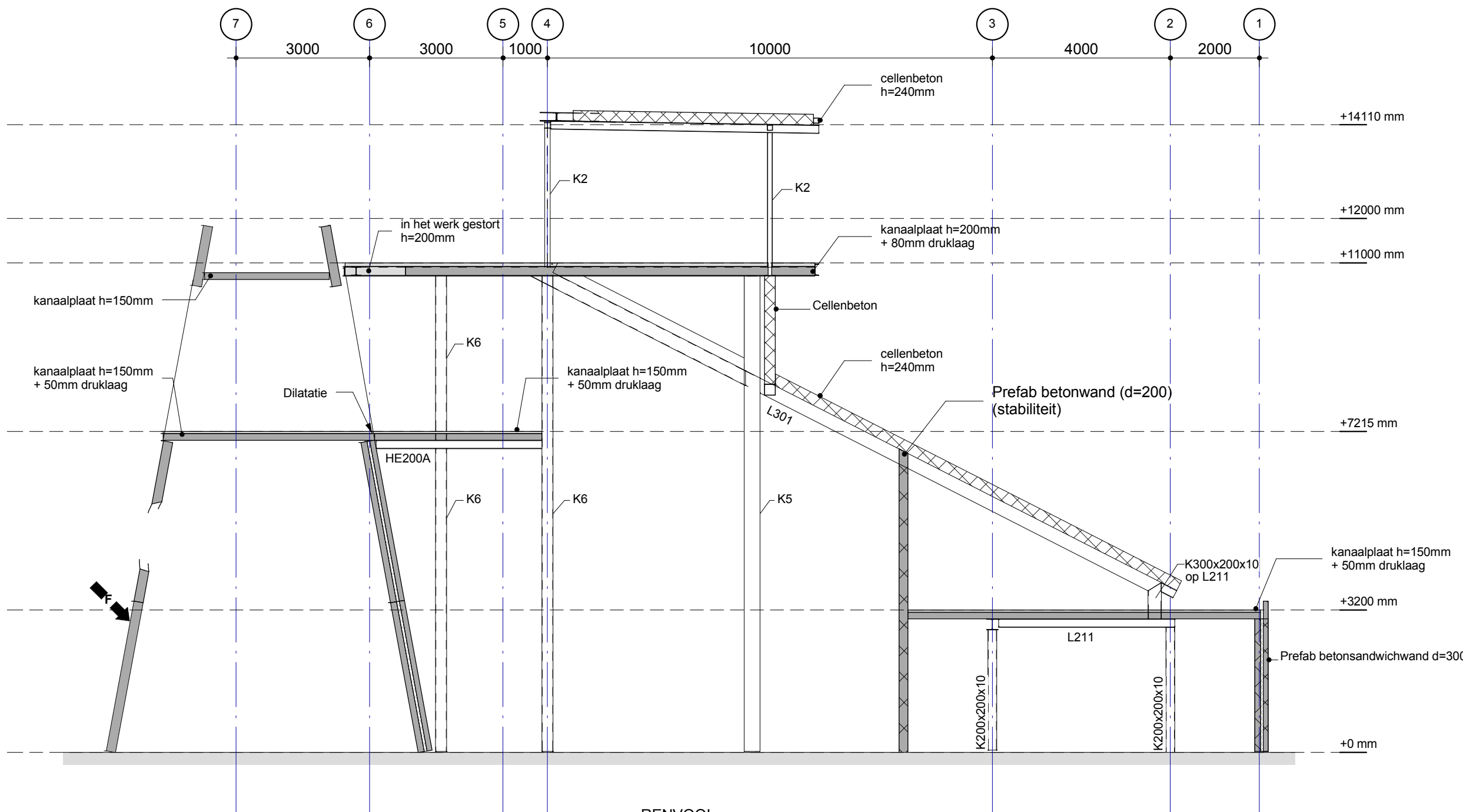
Doorsnede G-G
