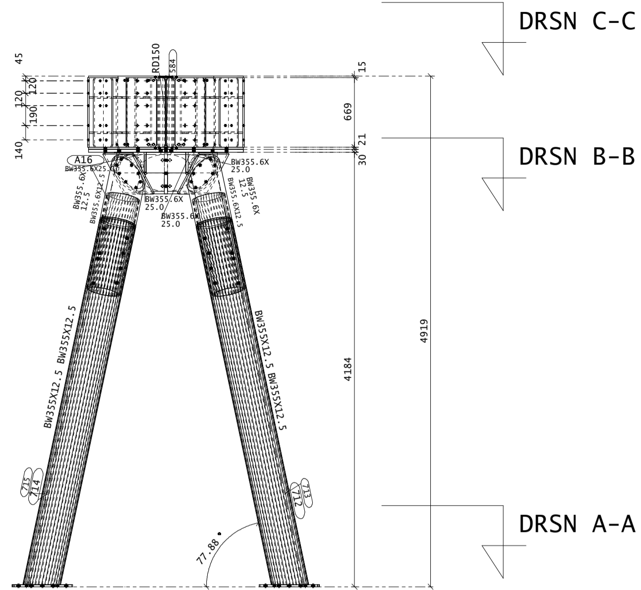
DOORSNEDE STATIEF SCHAAL 1:25
