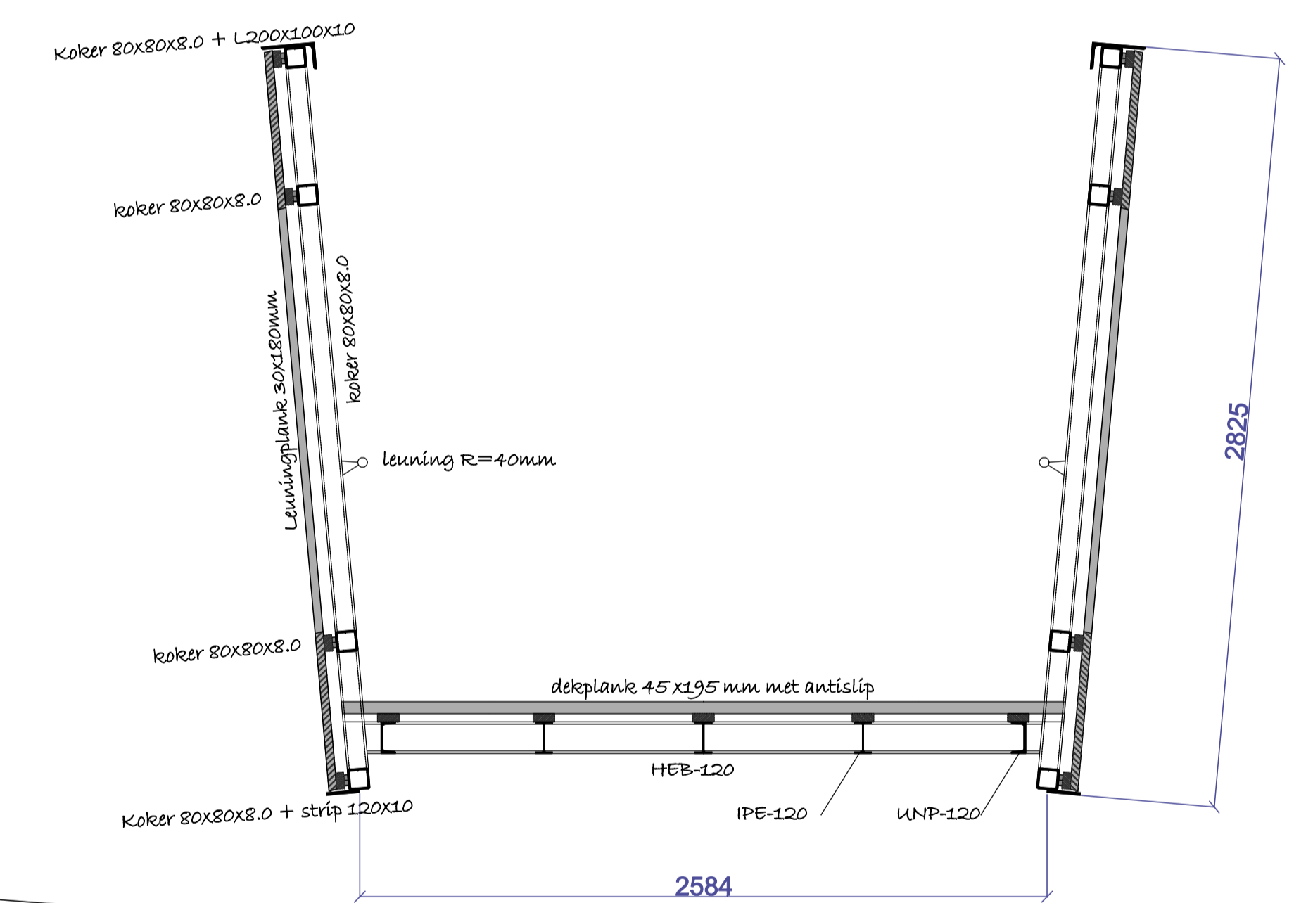
Dwars doorsnede
