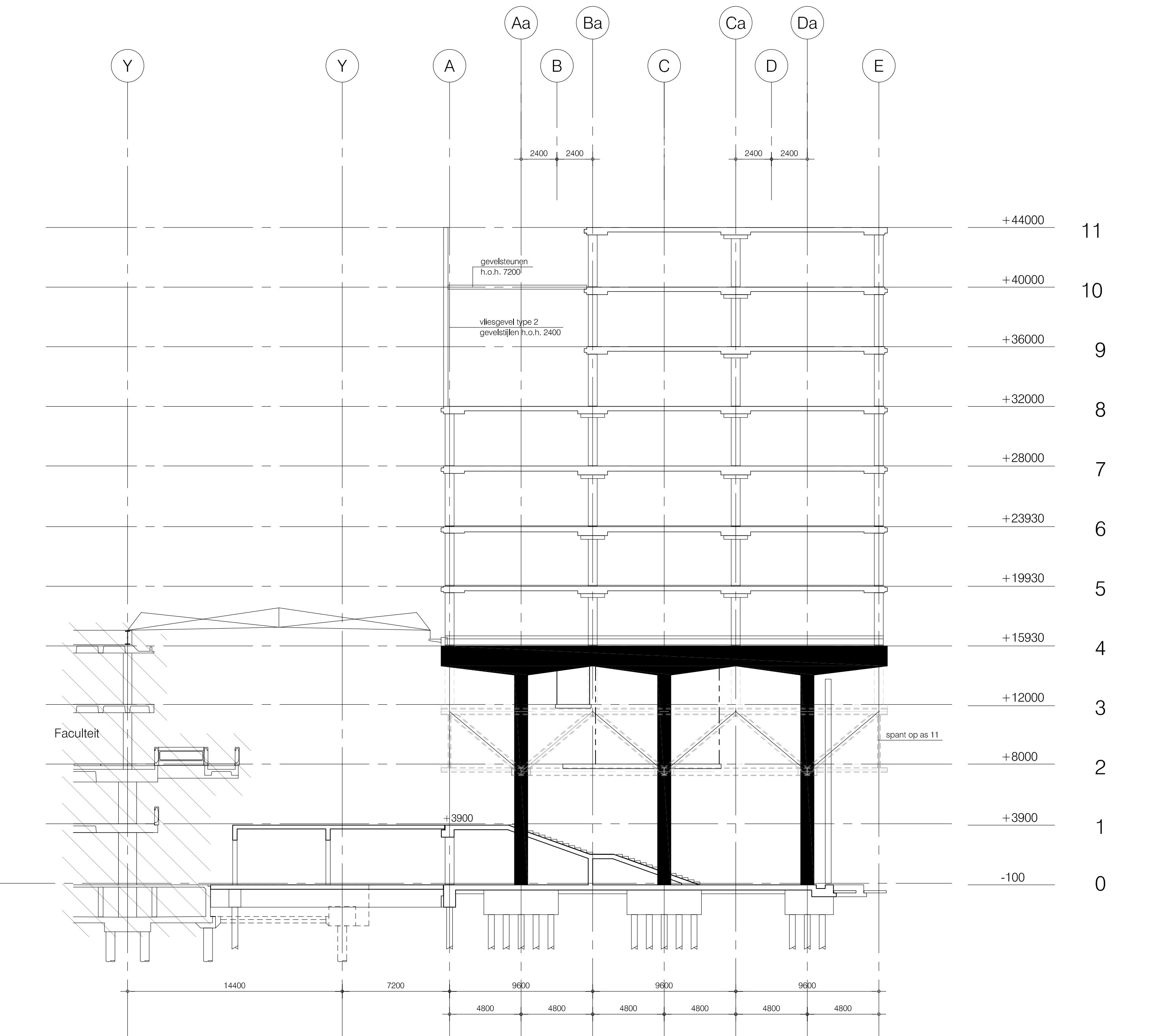
dwarsdoorsnede B-B tussen as 12 en 13
