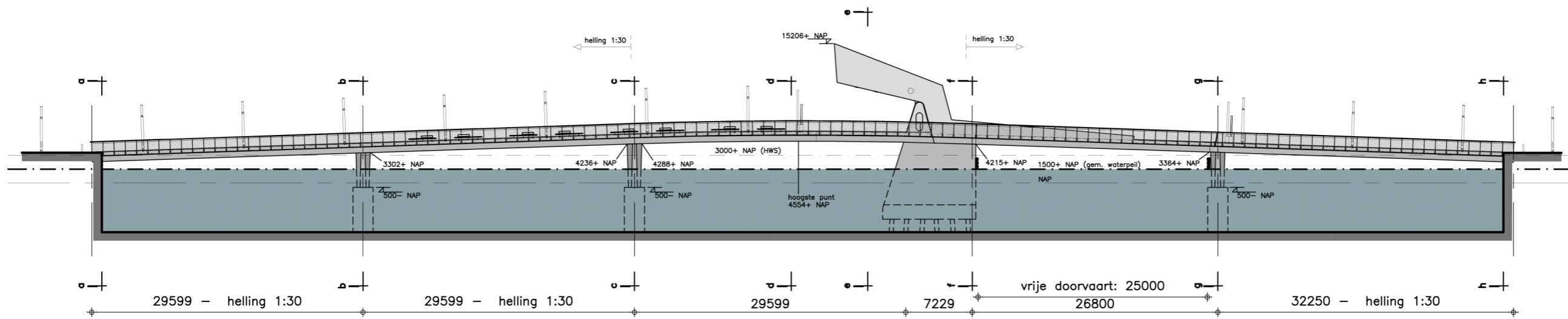
zijaanzicht schaal 1:500
