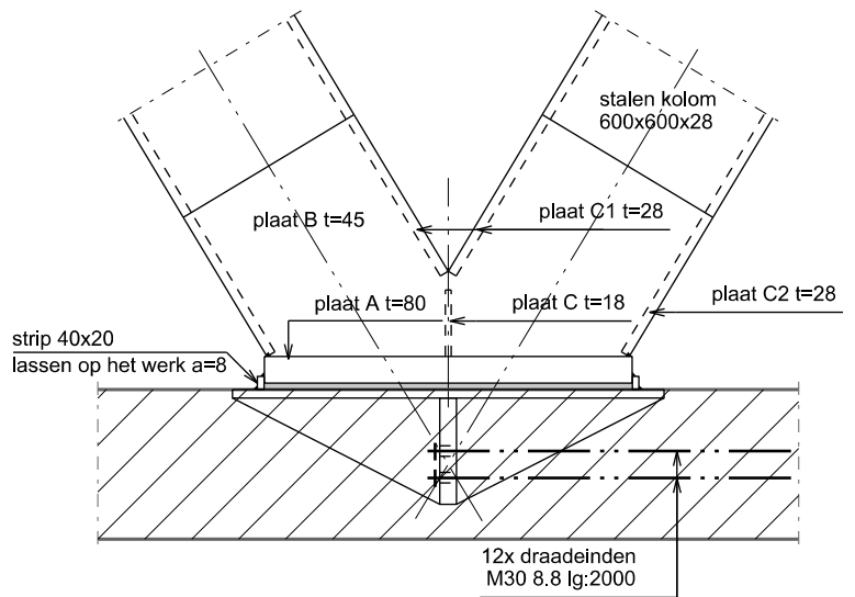
Aanzicht
