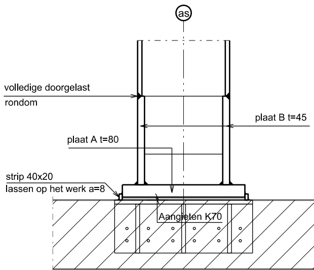
Doorsnede
