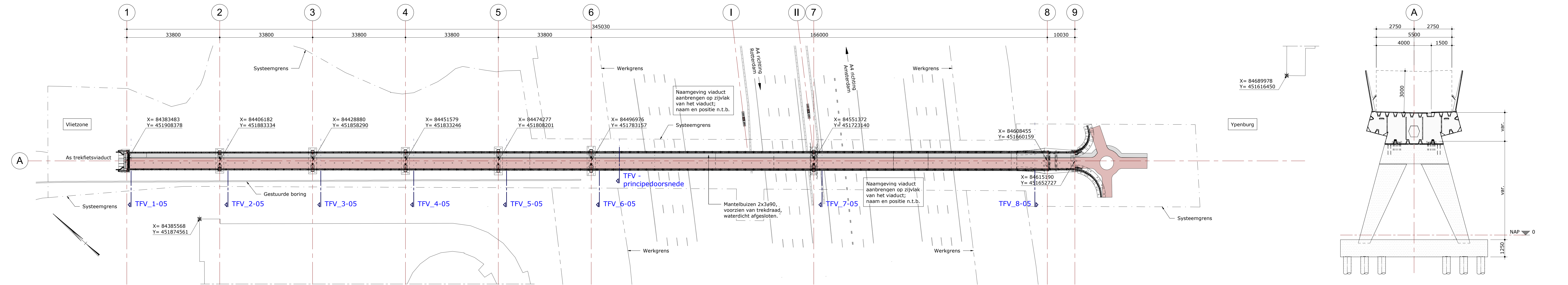
TFV - bovenaanzicht viaduct
