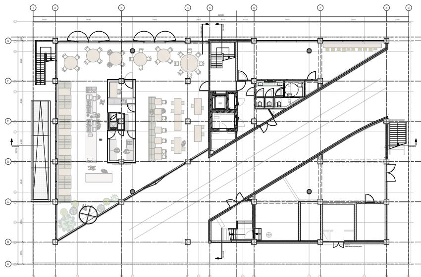
BEGANE GROND
