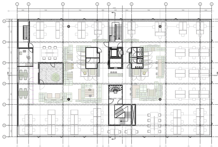
2E VERDIEPING
