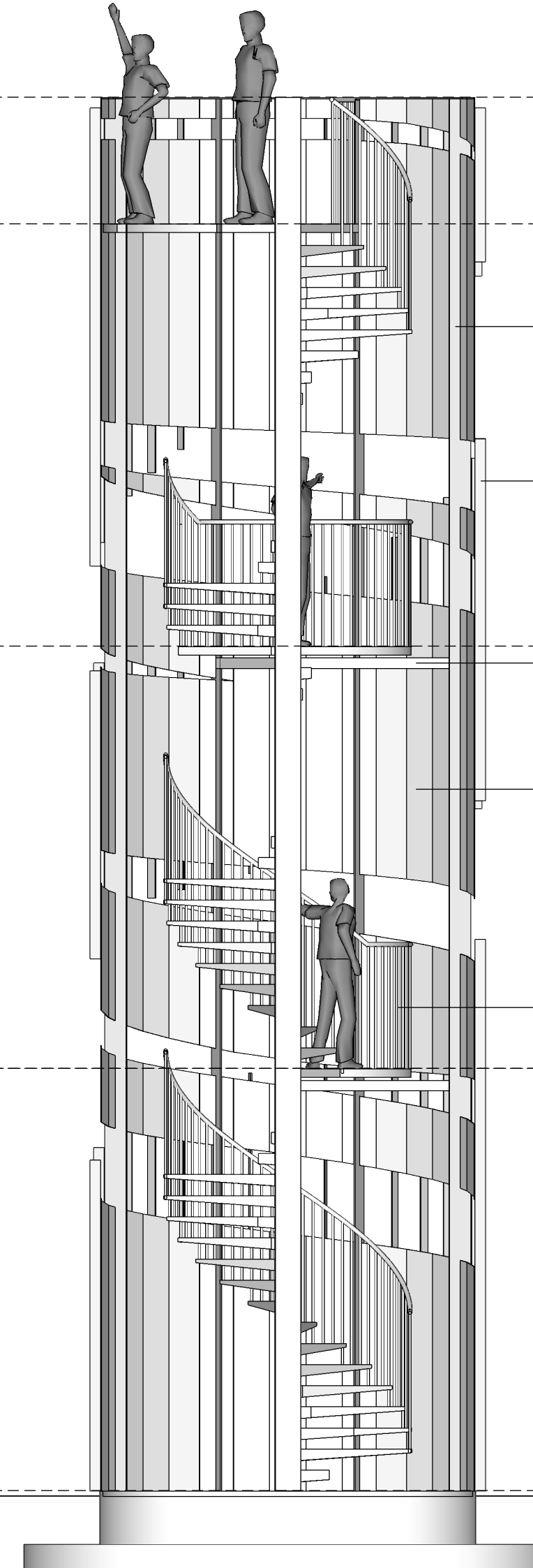
doorsnede B-B
