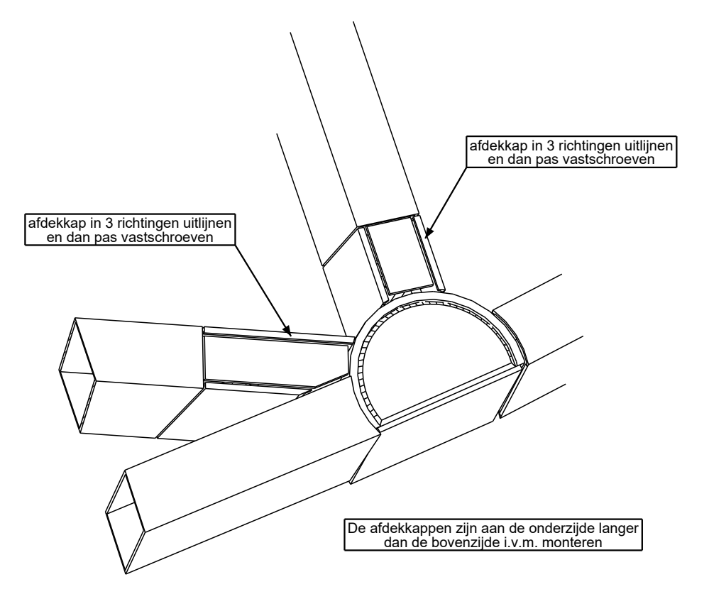
Algemeen detail (afdekkap) (met afdekkap en gelaste bovenplaat)
