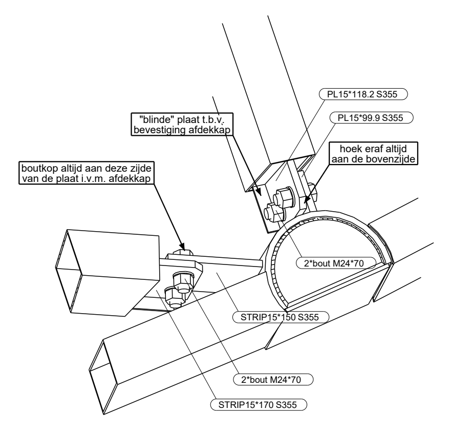
Algemeen detail (afdekkap) (zonder afdekkap en gelaste bovenplaat)
