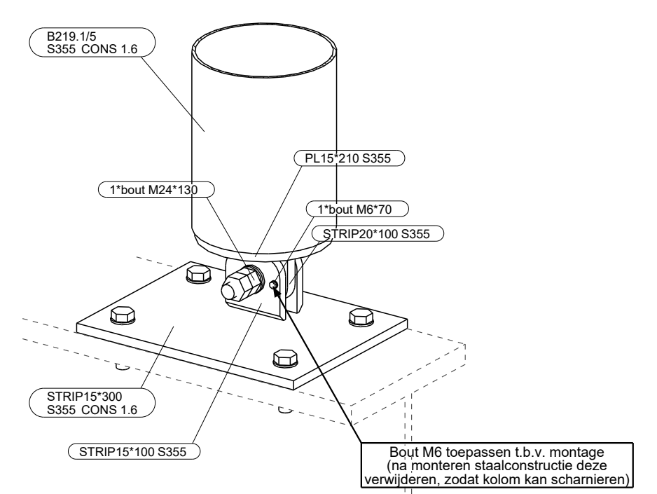
Algemeen detail (kolomaansluiting onderzijde)
