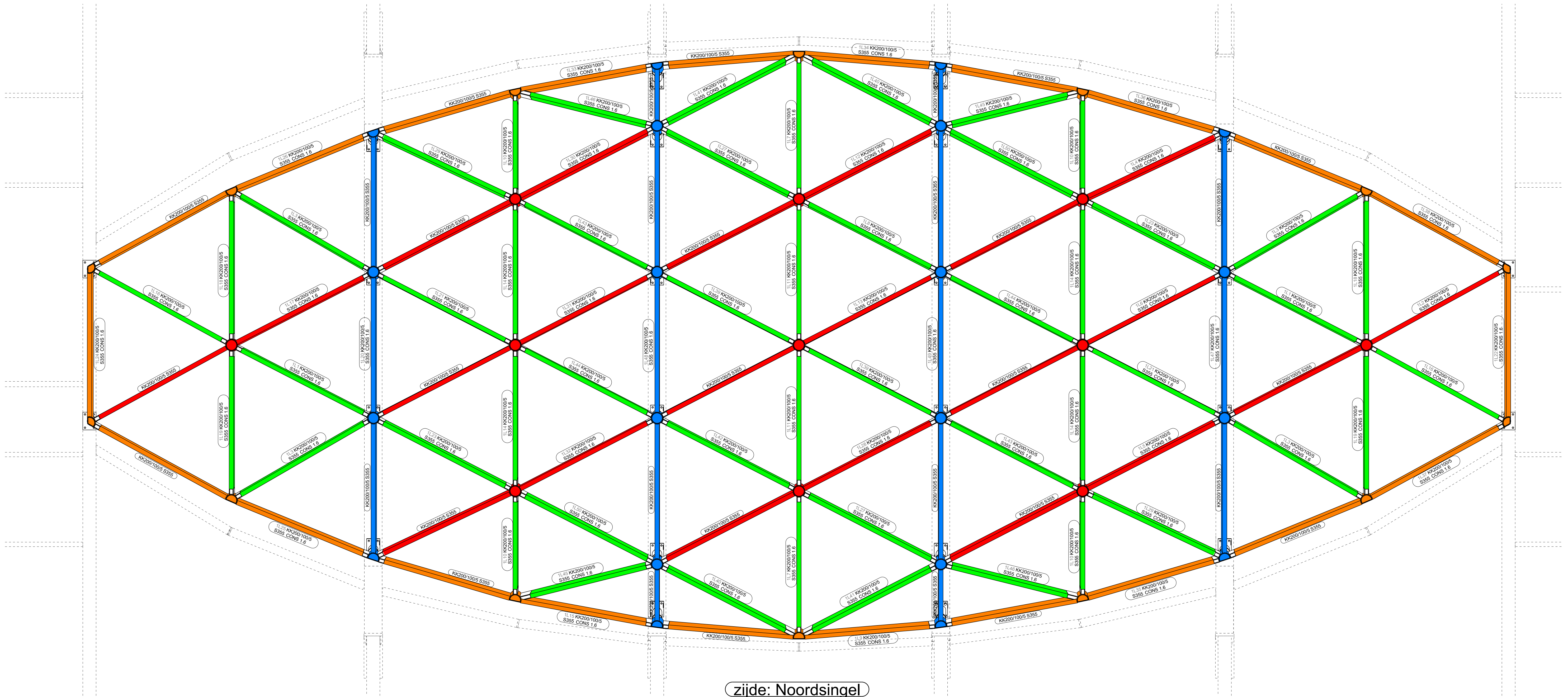
Bovenaanzicht, 1:45 (in kleur aangegeven doorlopende liggers)
