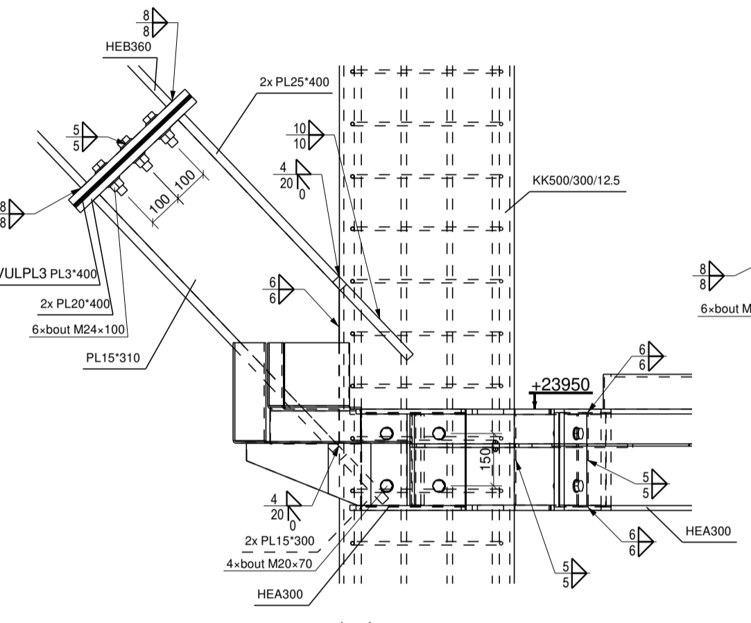
detail 1, 1:15
