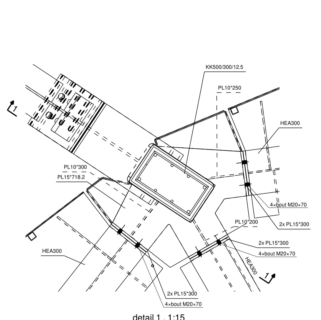
detail 1, 1:15
