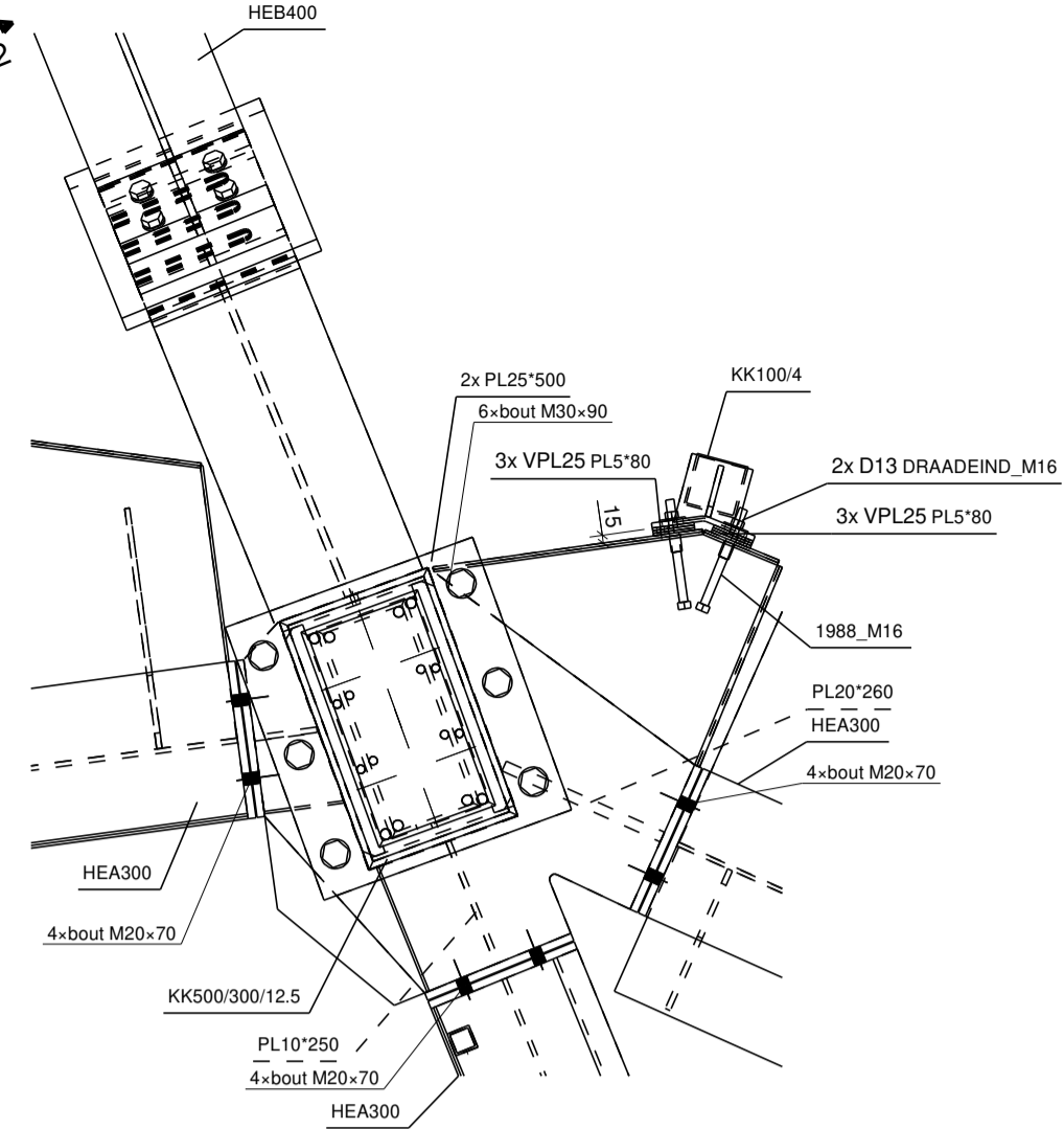
detail 2, 1:15
