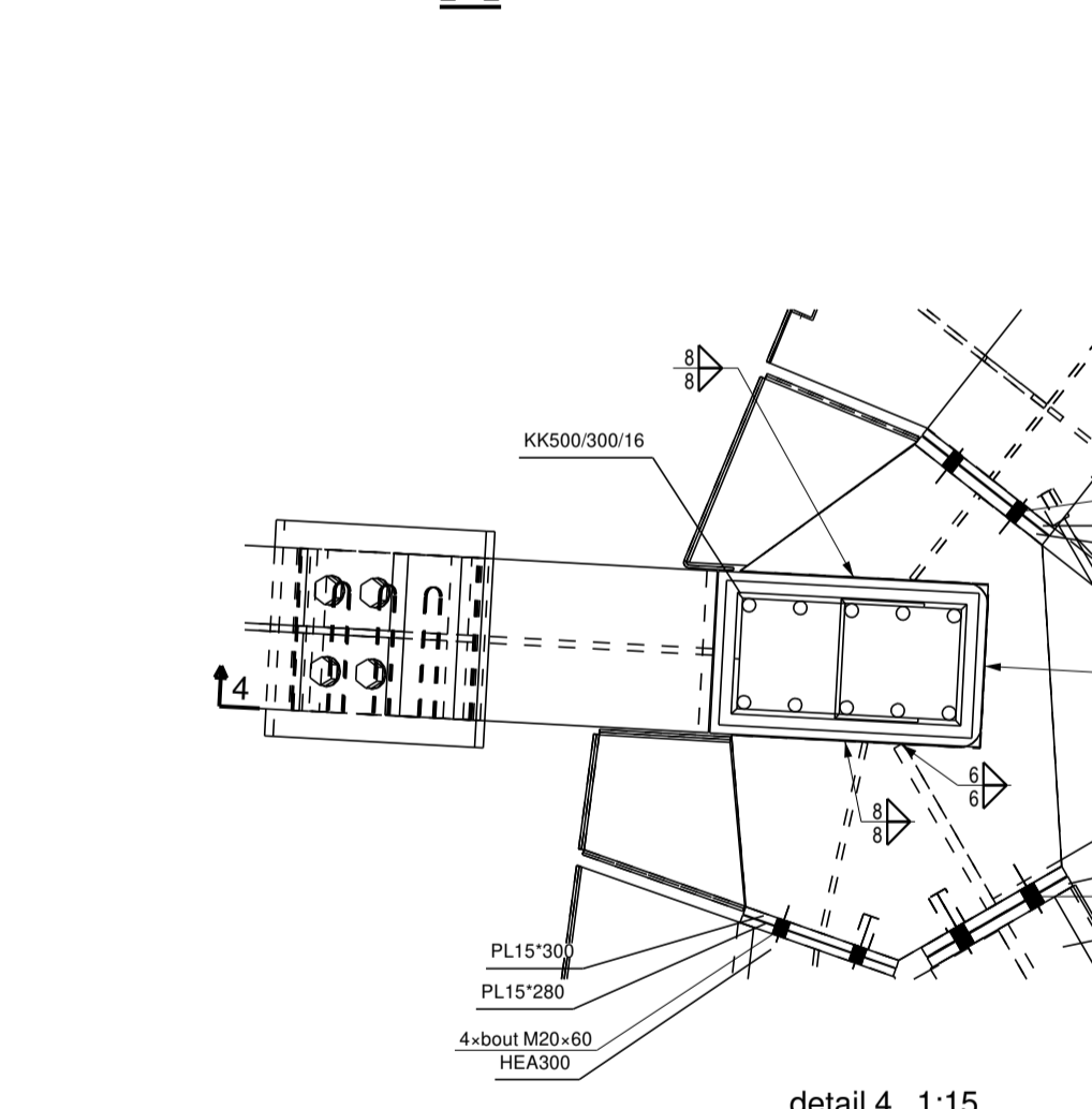
detail 4, 1:15
