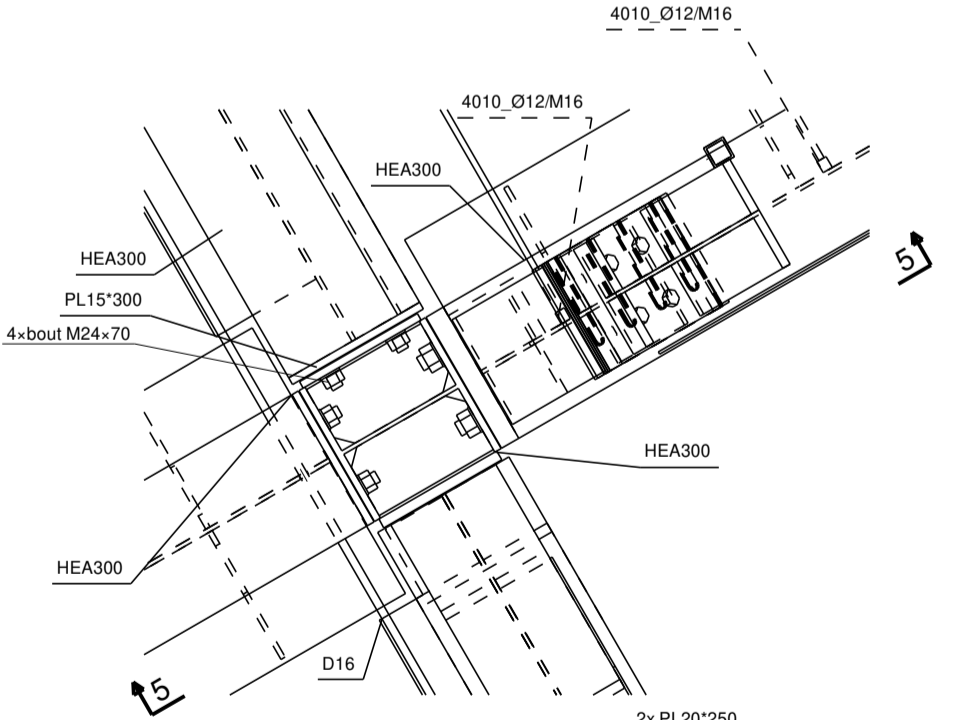
detail 5, 1:15
