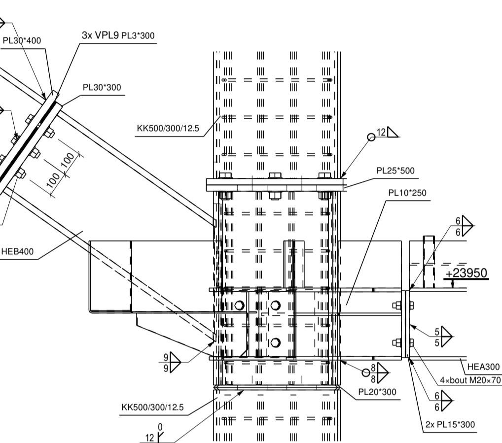
detail 2, 1:15
