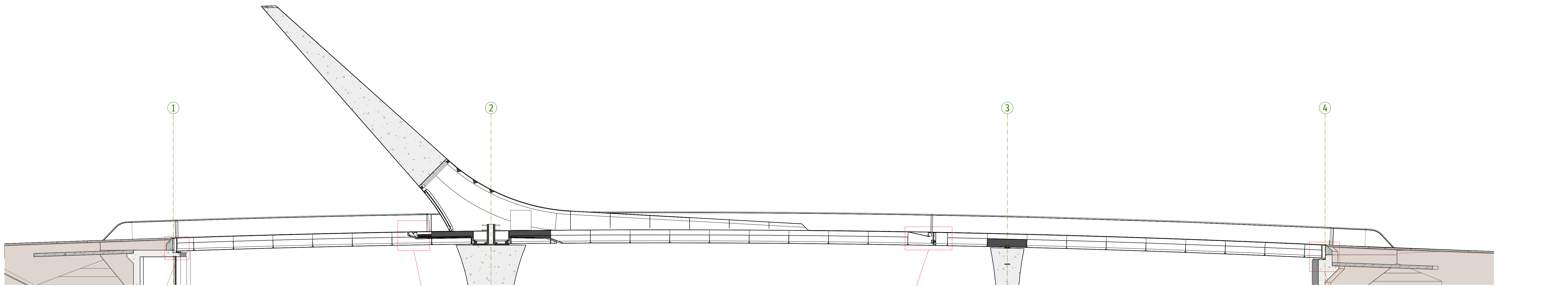
LANGSDOORSNEDE BRUGDEK SCHAAL 1:100
