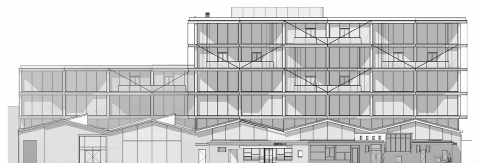
↑ TEKENING VAN DE OOSTGEVEL
