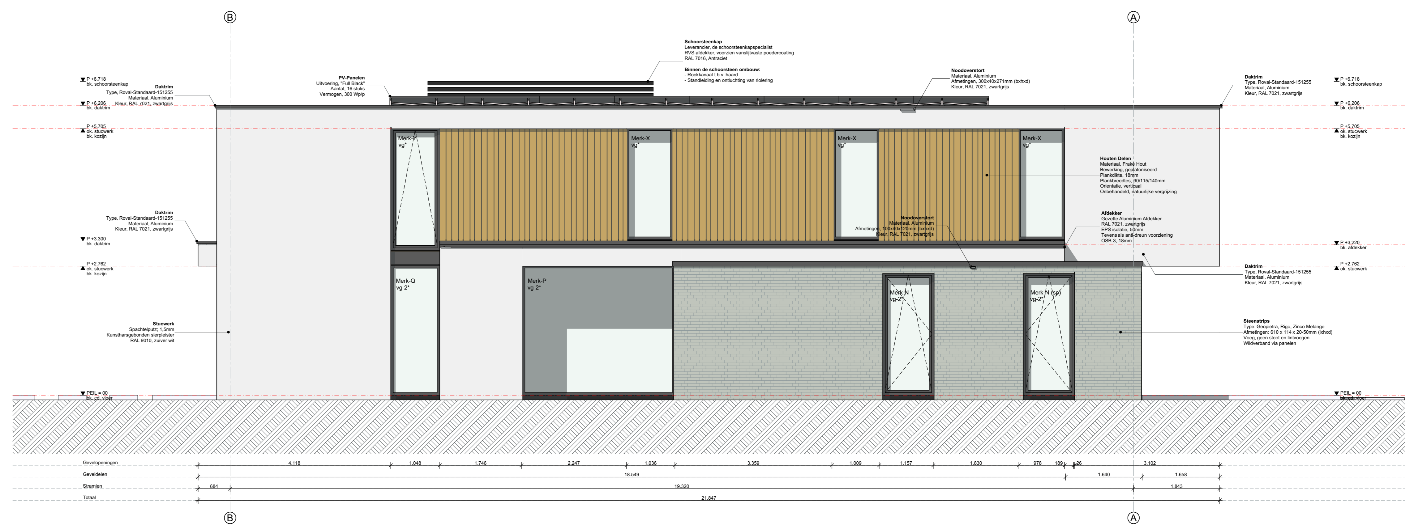
Rechtergevel
