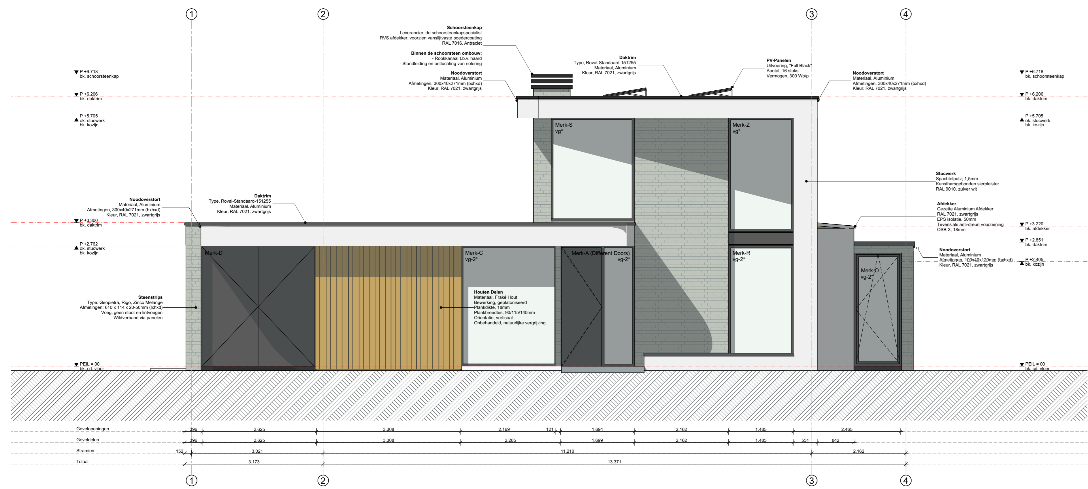
Voorgevel
