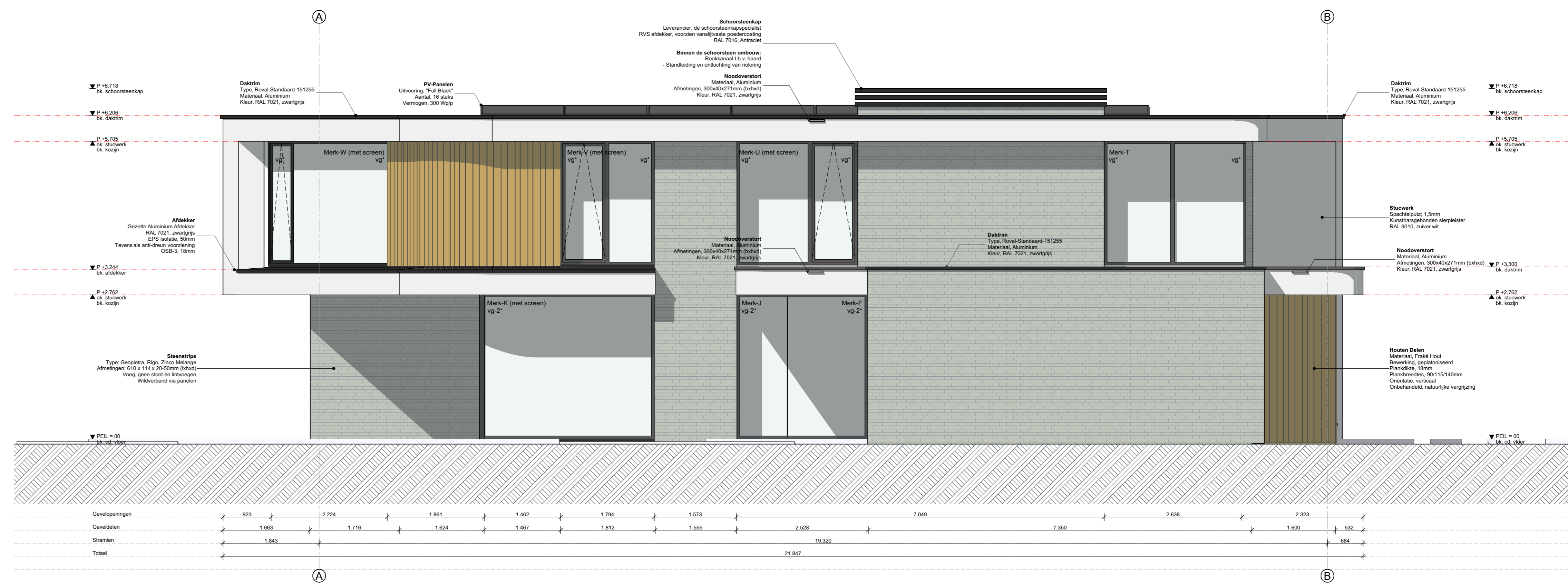
Linkergevel
