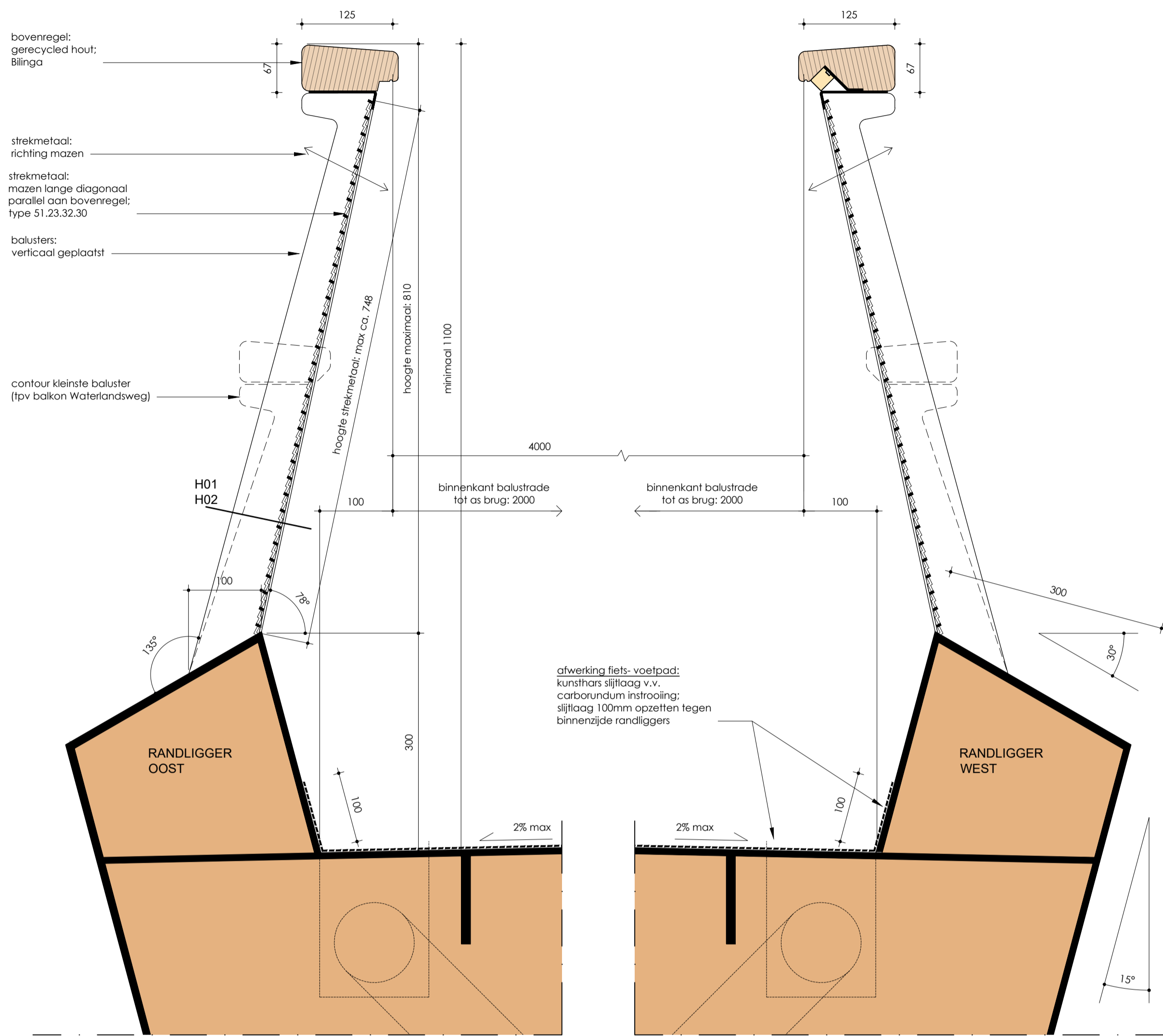
standaard baluster oostzijde schaal 1:5
