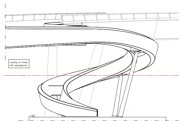
Zijaanzicht Noord-Zuid schaal: 1:50
