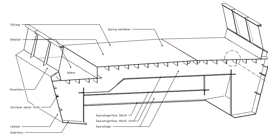
DWARSDOORSNEDEN DEK (GESLOTEN EN OPEN)
