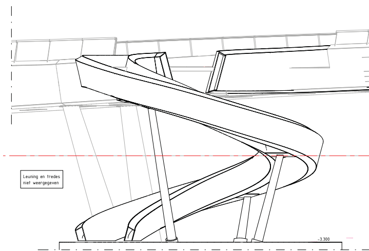
Zijaanzicht West-Oost schaal: 1:50
