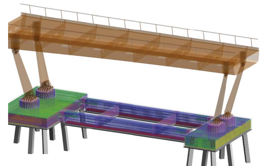
3D DOORSNEDE STEUNPUNT
