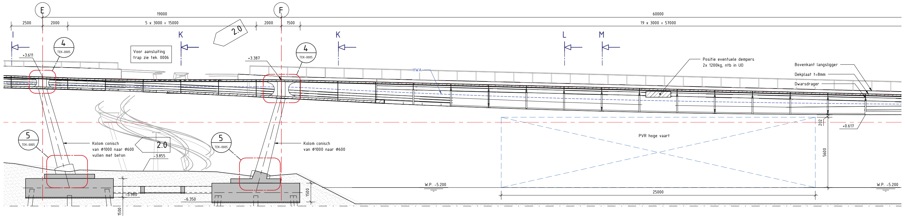
LANGSDOORSNEDE 3
