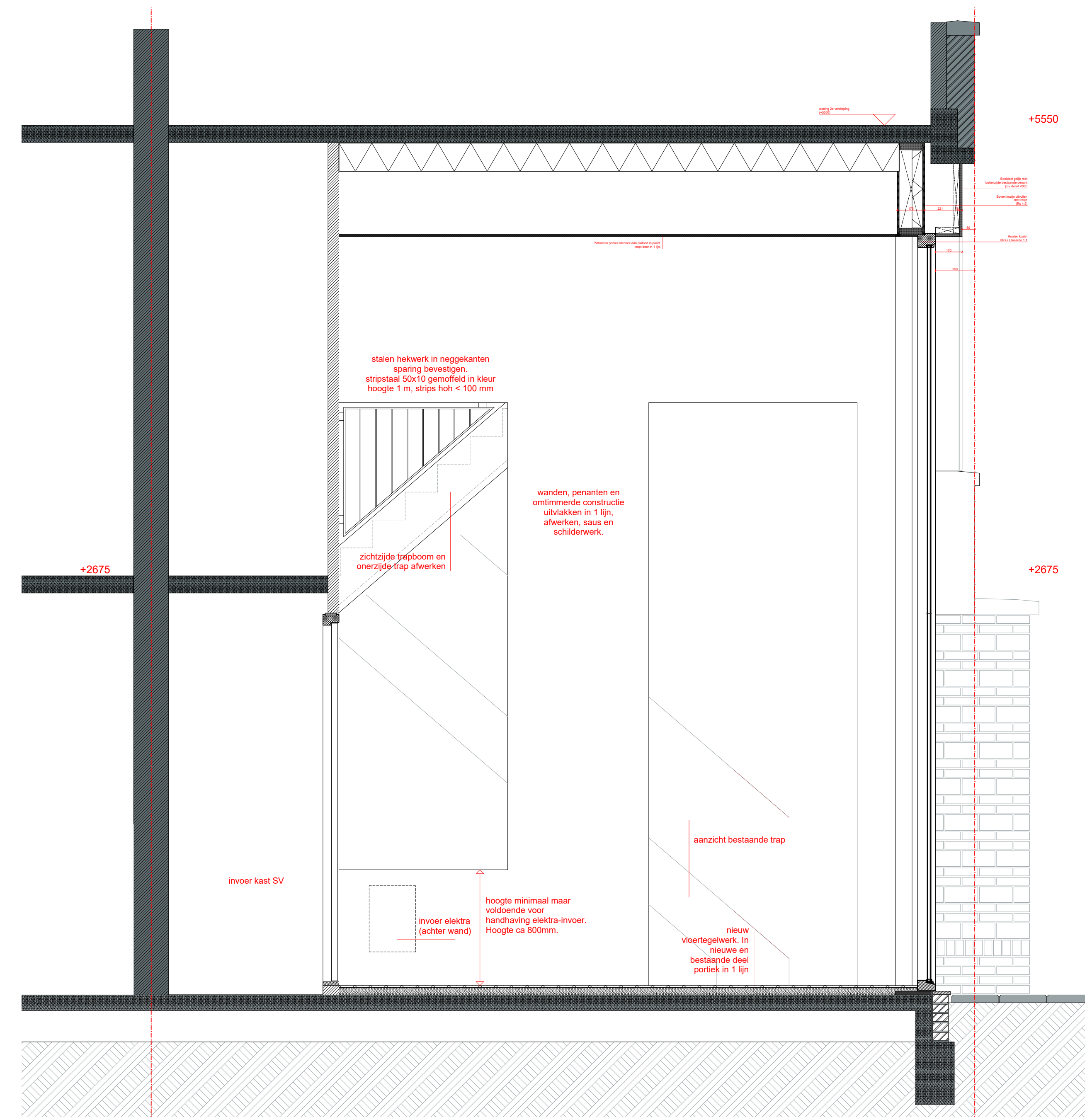
DOORSNEDE CC2
