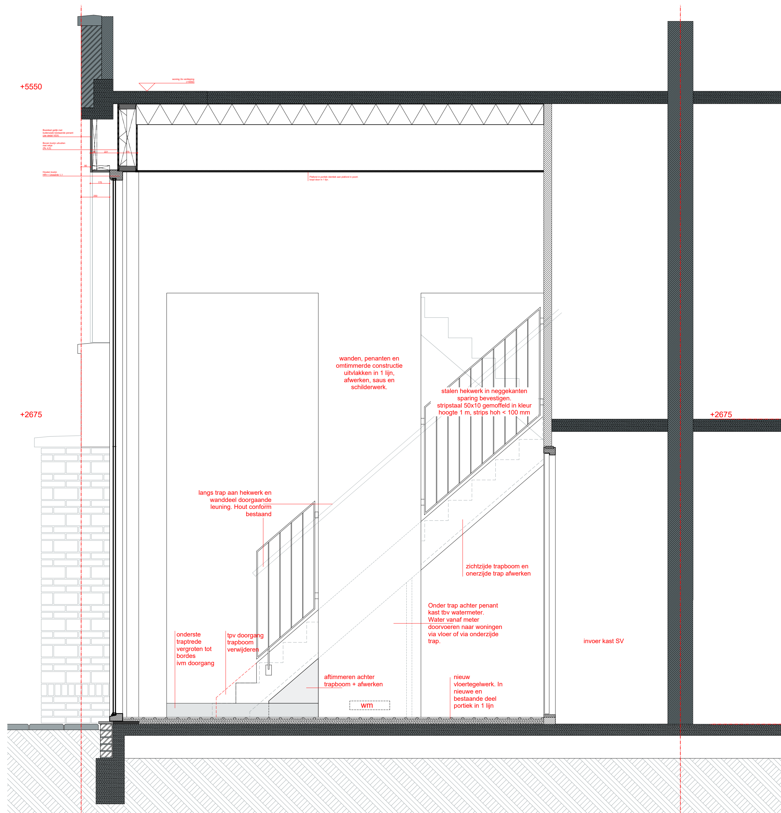
DOORSNEDE CC1
