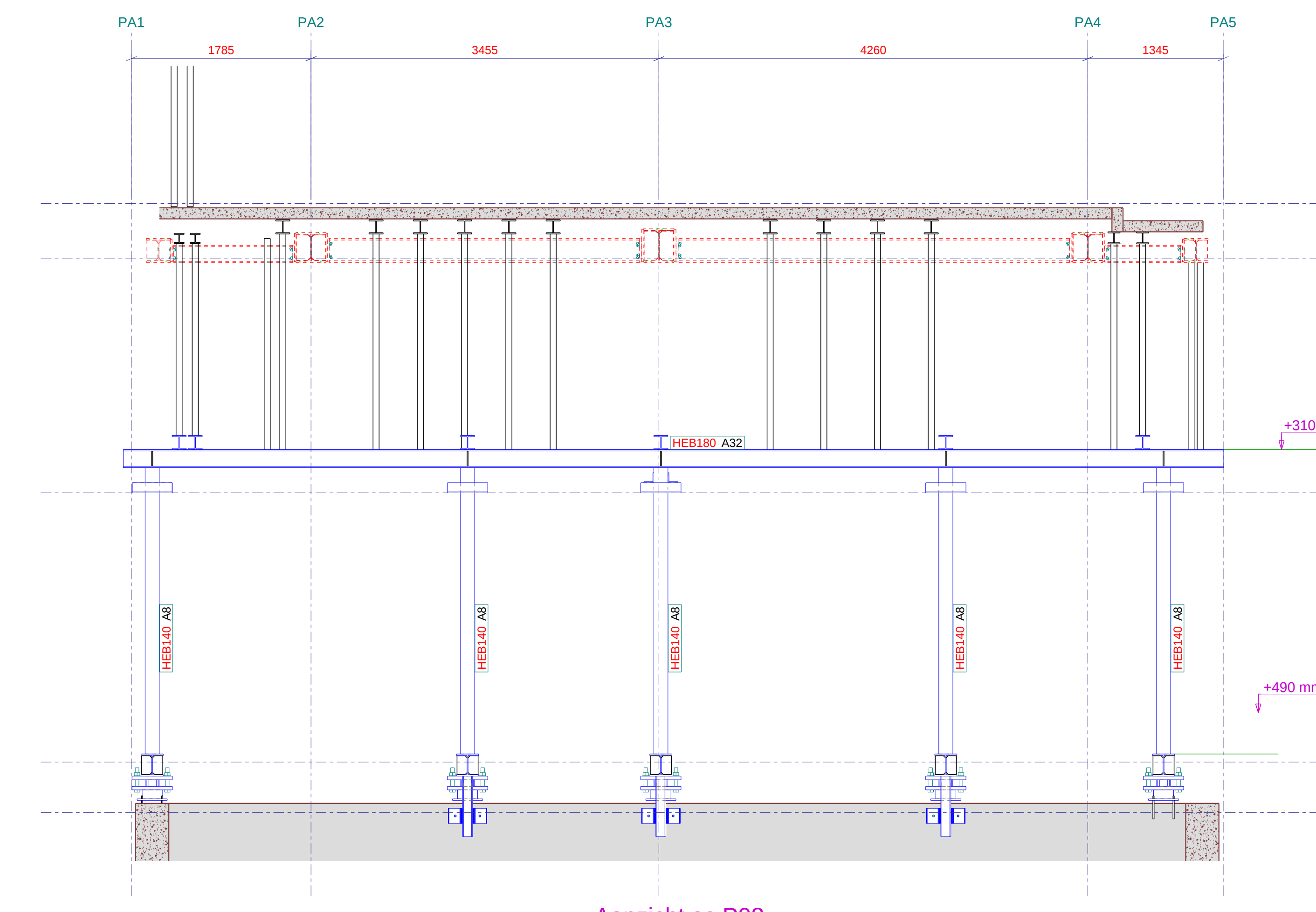
Aanzicht as P08 1:35
