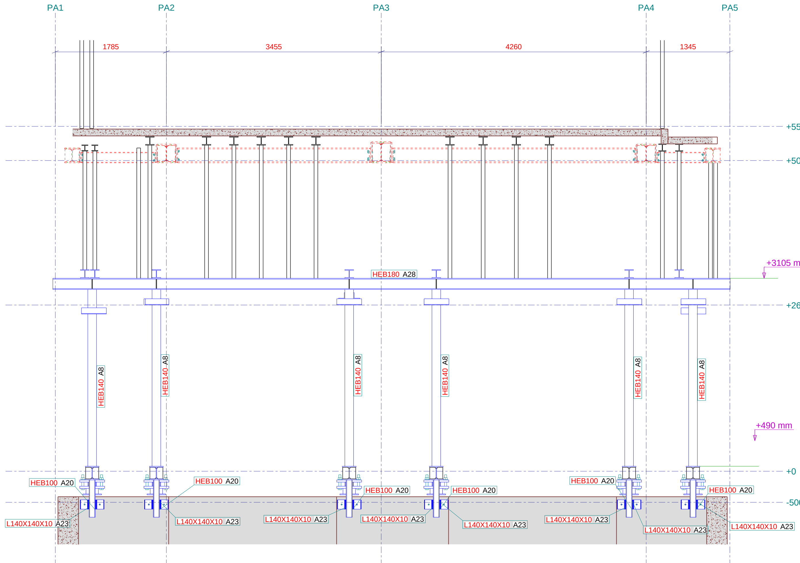
Aanzicht as P06 1:35
