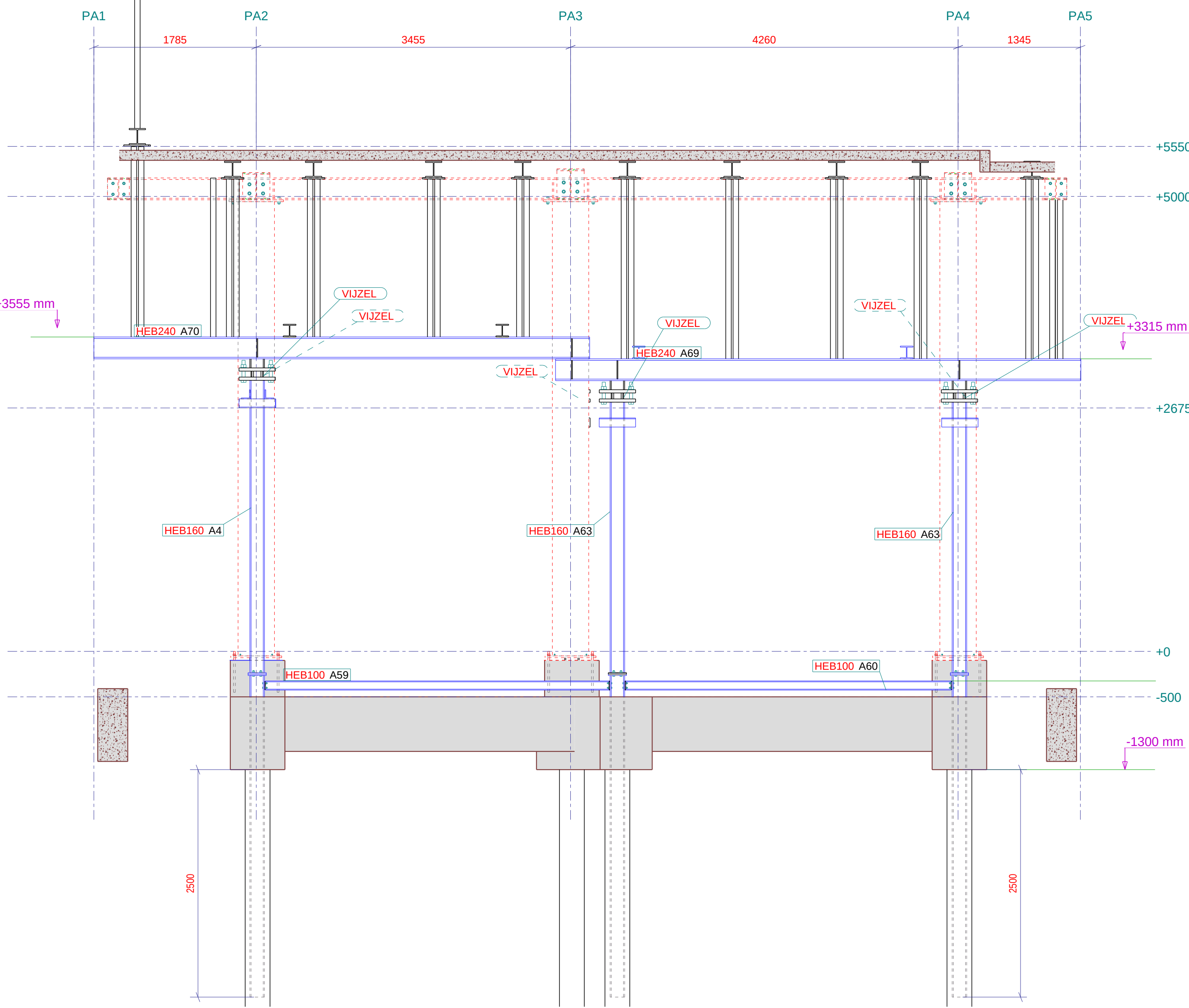
Aanzicht as P07a 1:35
