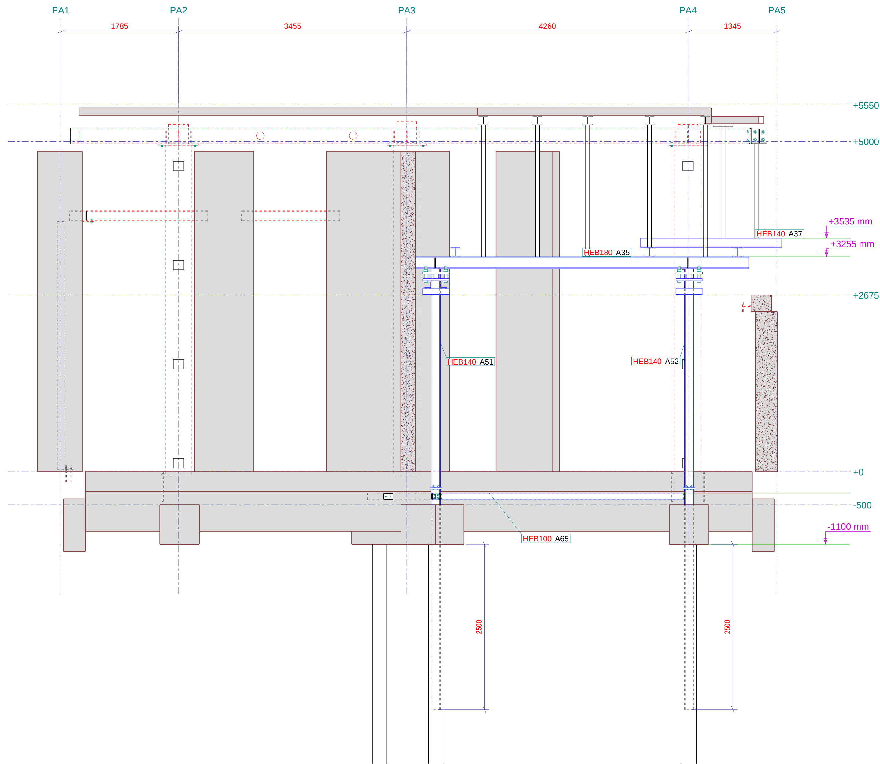
Aanzicht as P09 1:35
