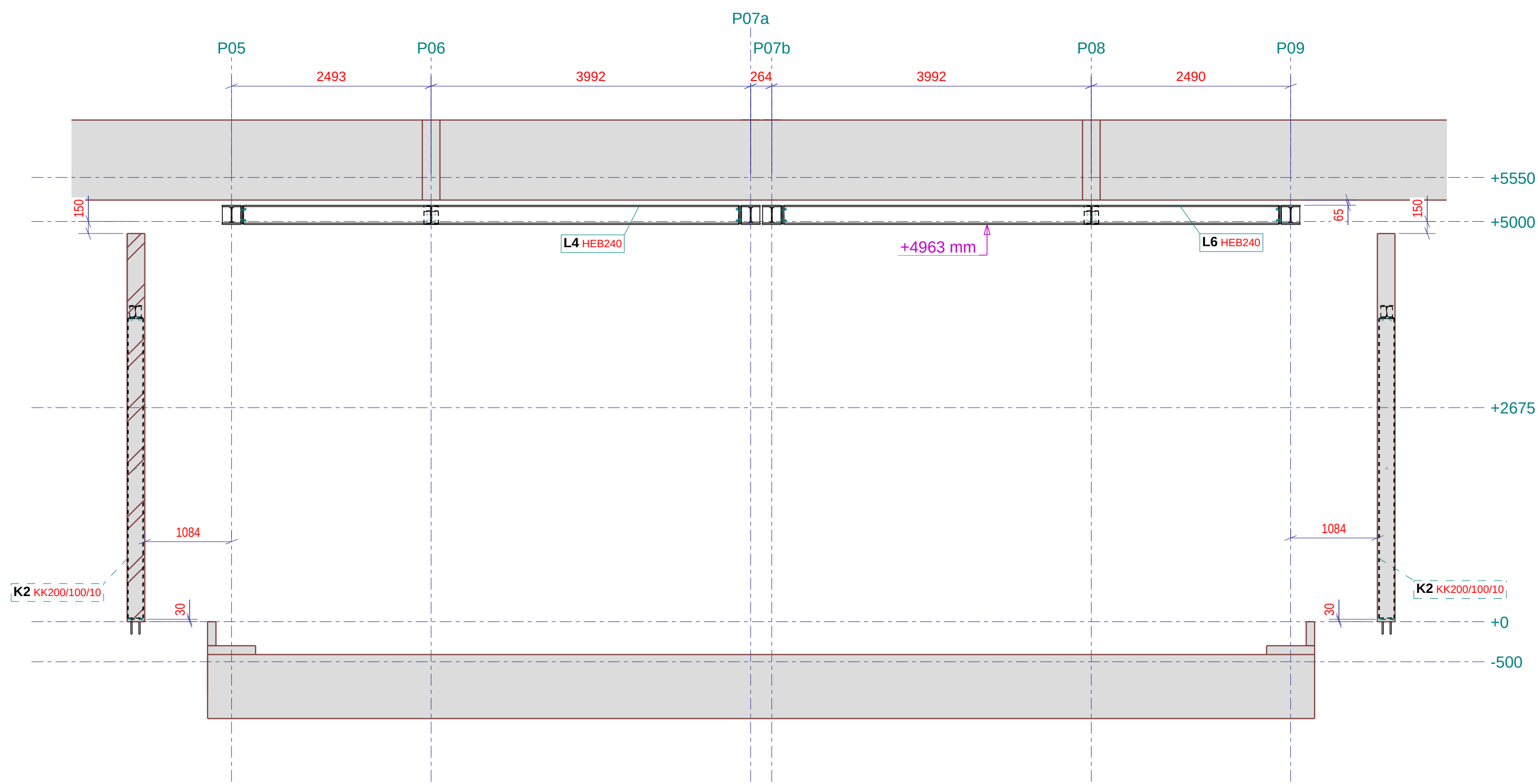
Aanzicht as PA1 1:50
