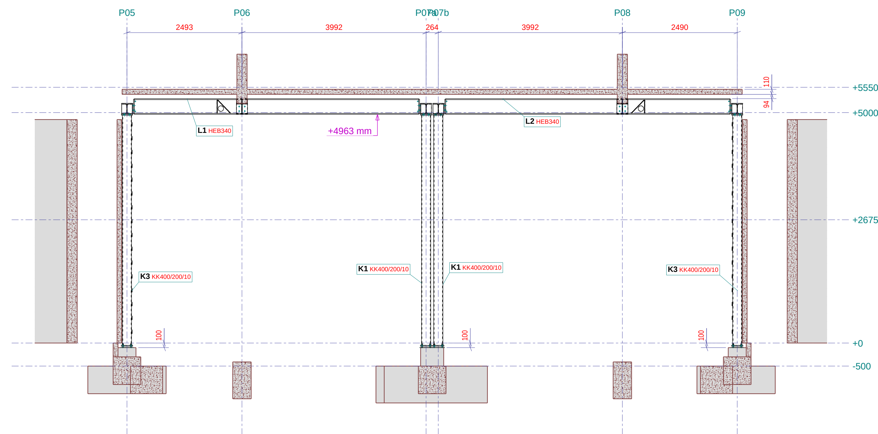
Aanzicht as PA3 1:50
