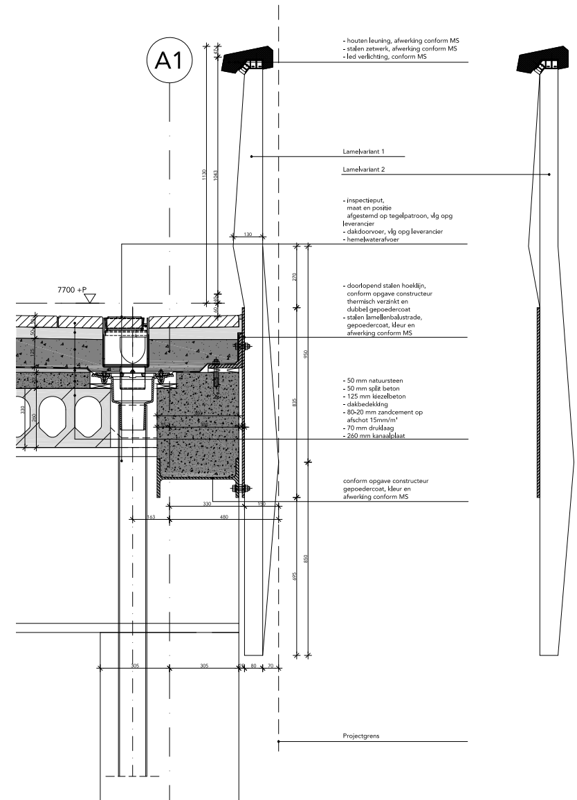
Detailtekening opbouw en bevestiging stalen lamellenbalustrade.
