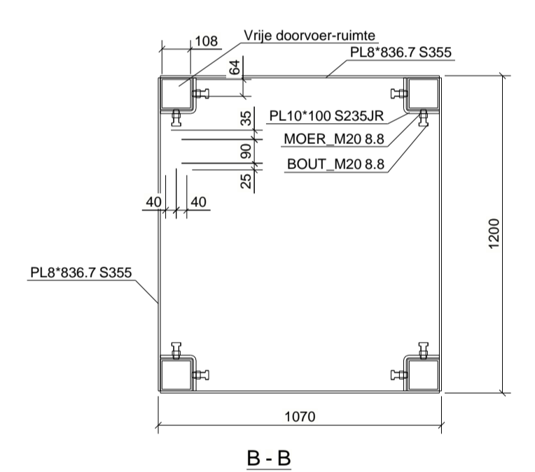
B - B
