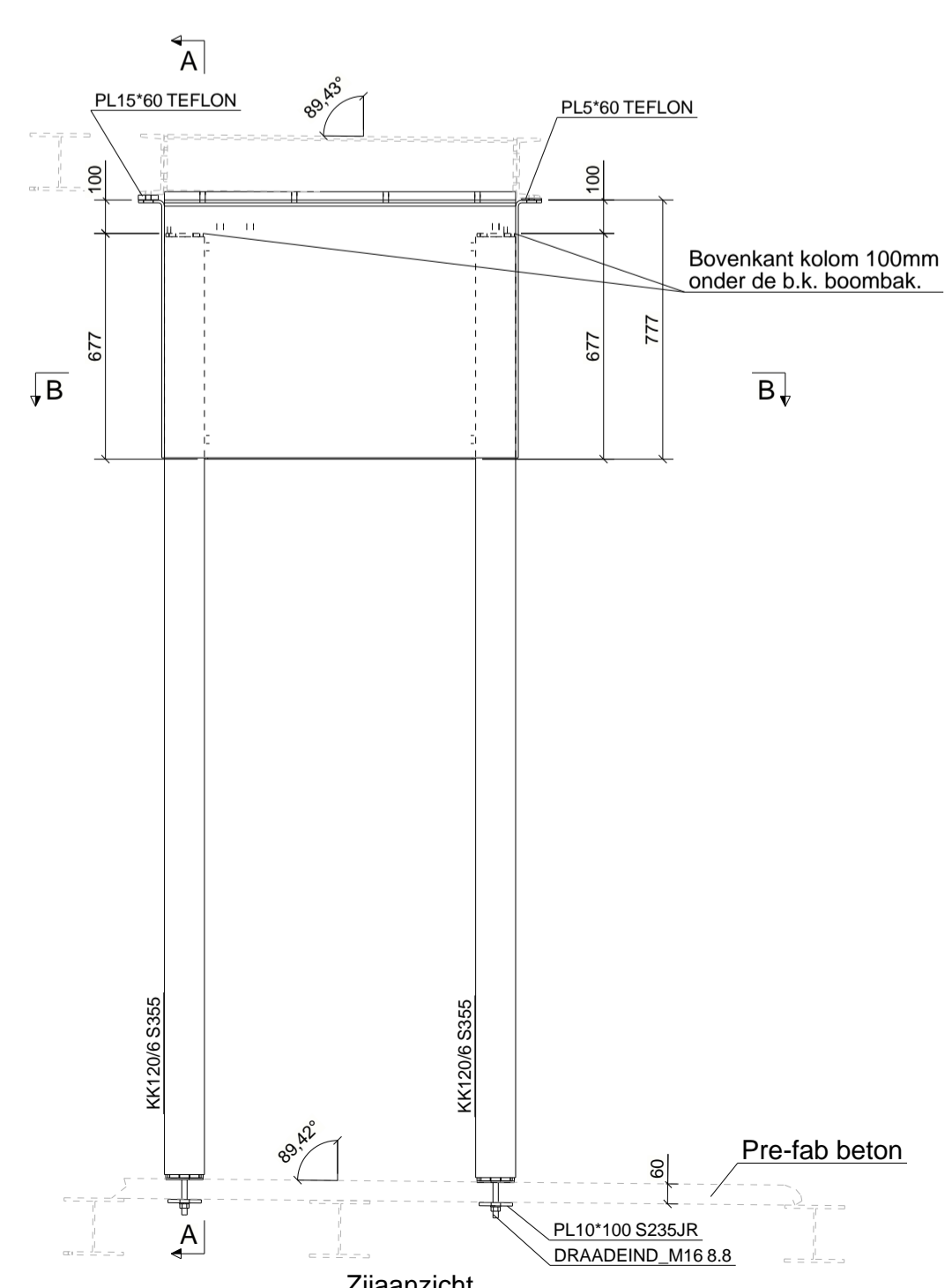
Zijaanzicht
