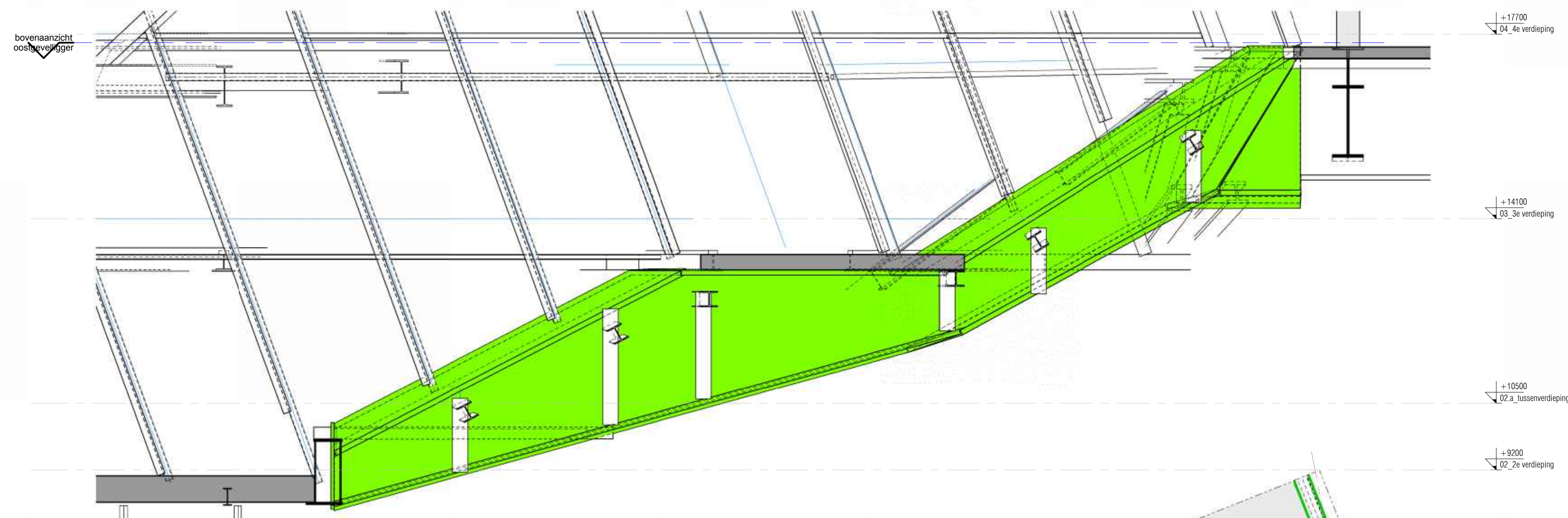
aanzicht trap-ligger 1 : 50
