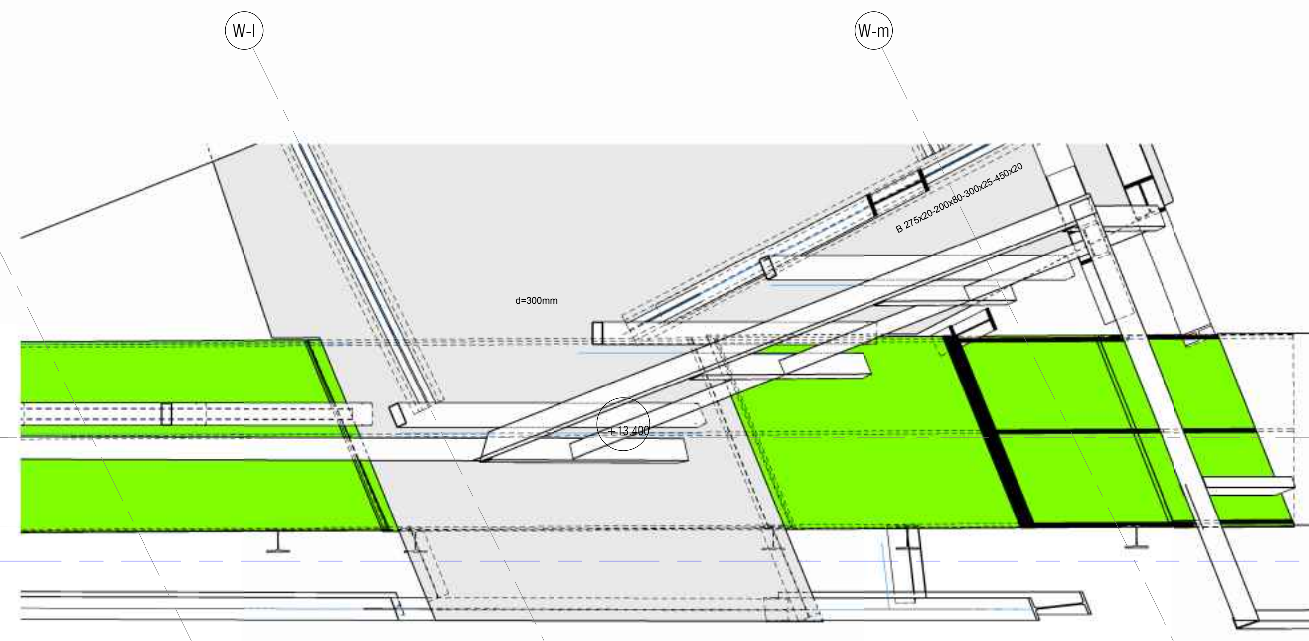
03_3e verdieping trap-ligger 1 : 50
