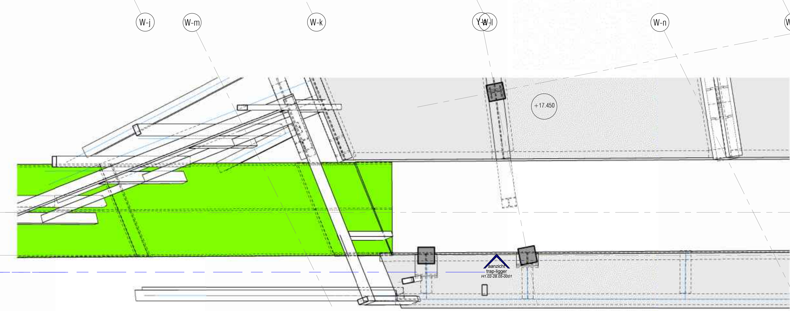
bovenaanzicht oostgevelligger 1 : 50
