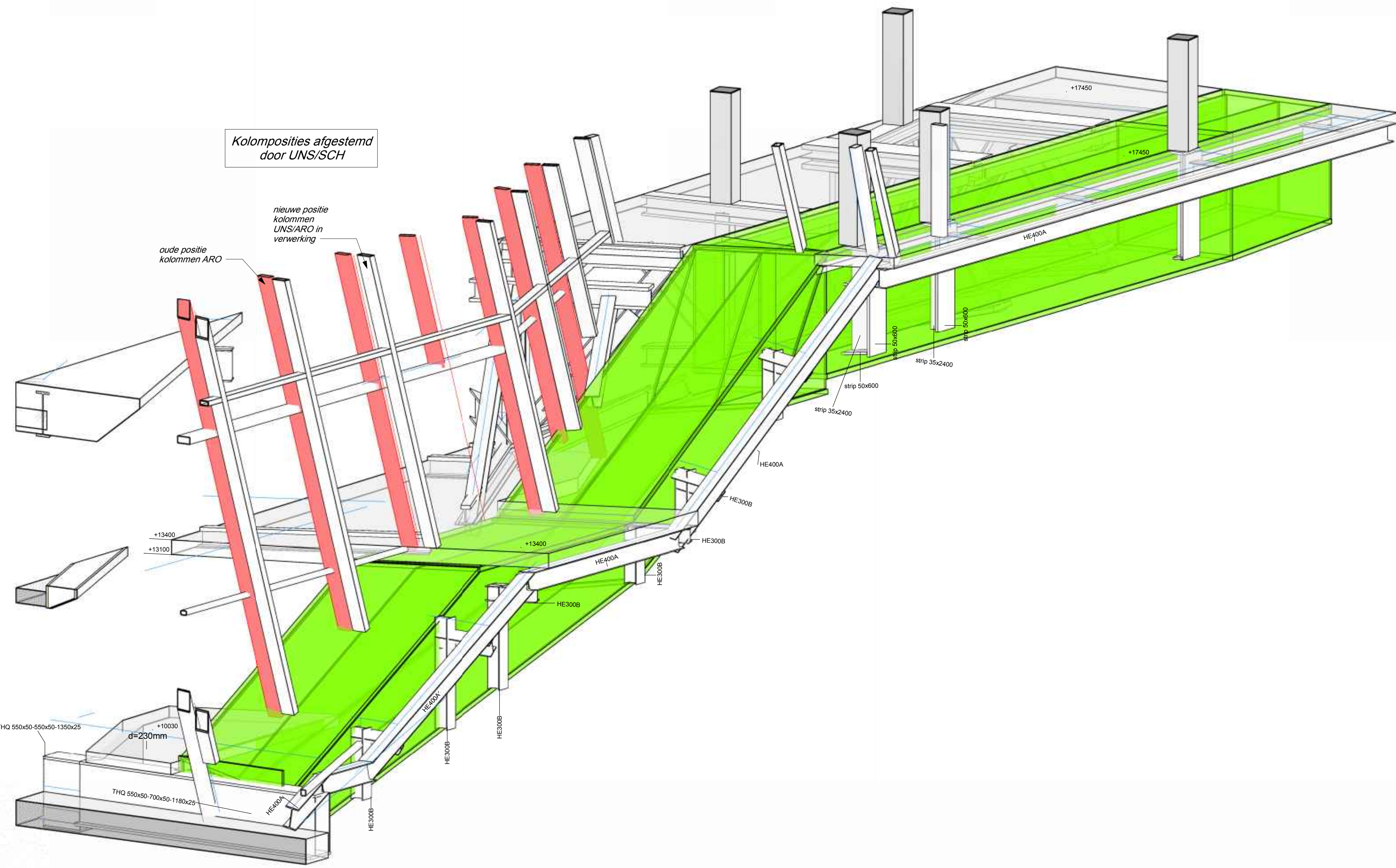
overzicht spanten tpv liften
