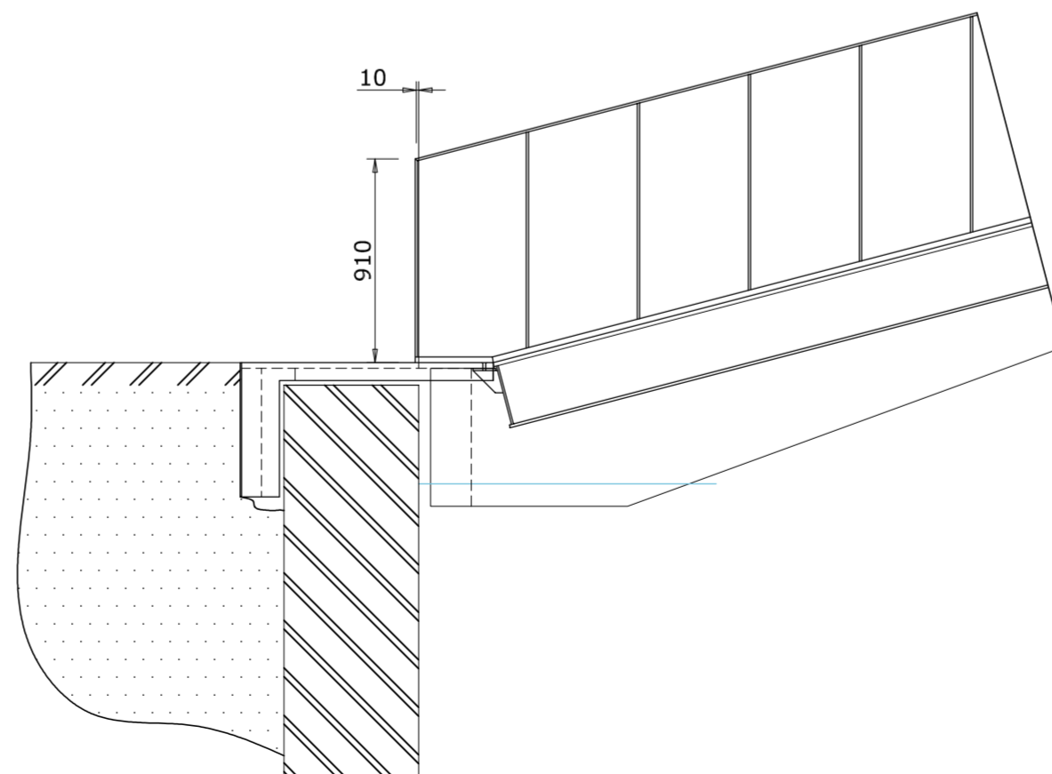
Aanzicht A-A - optie 2 1:30
