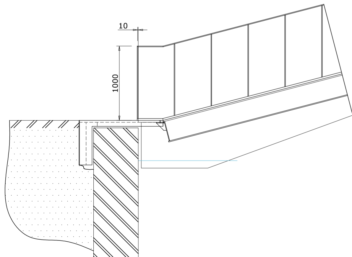
Aanzicht A-A - optie 1 1:30
