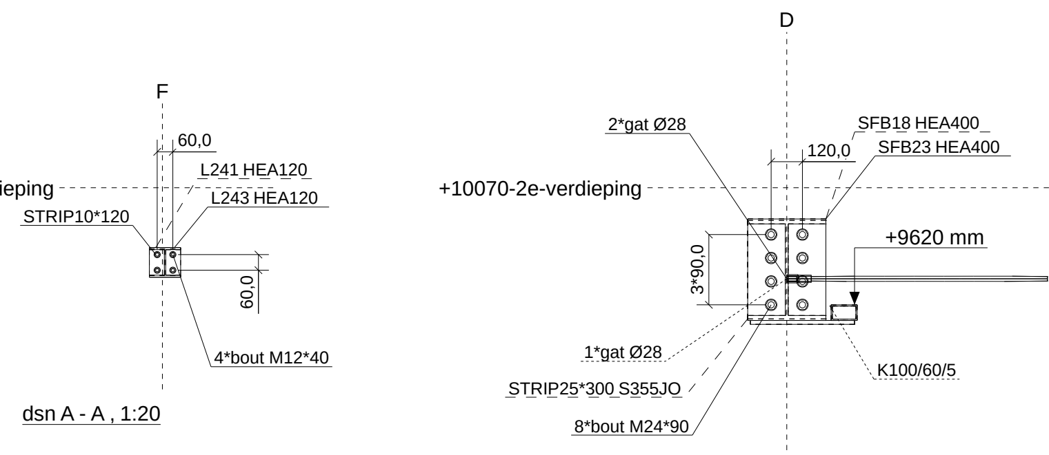
dsn B - B, 1:20
