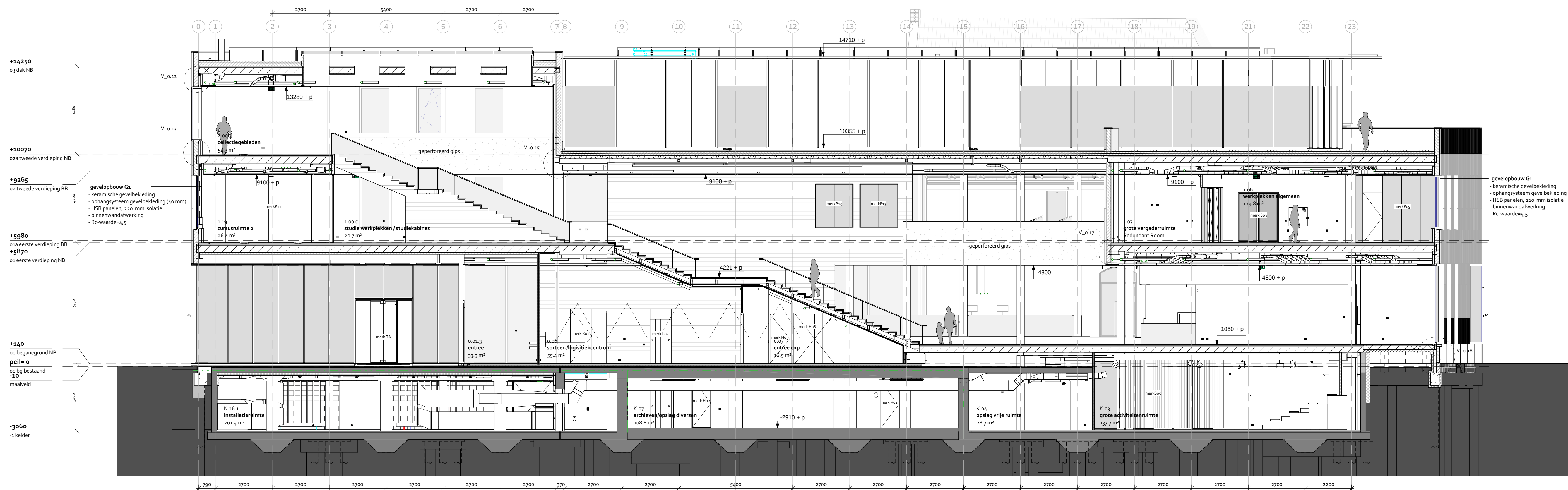
Doorsnede A-A
