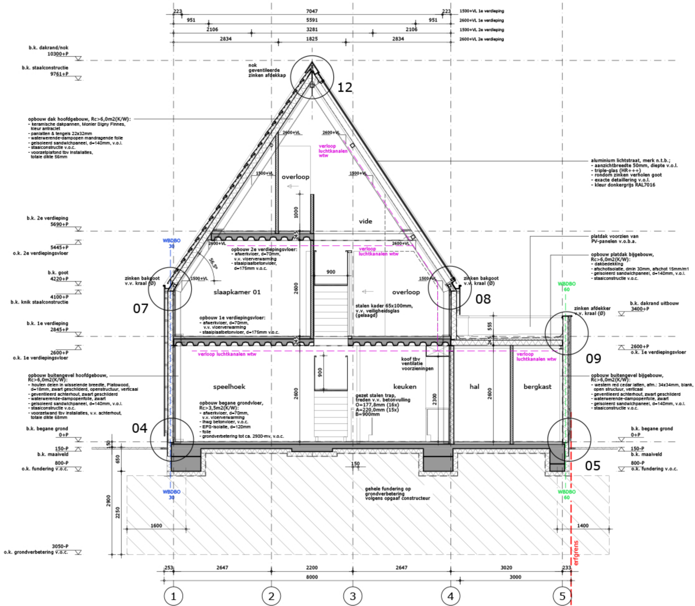
Doorsnede A-A Schaal 1:50
