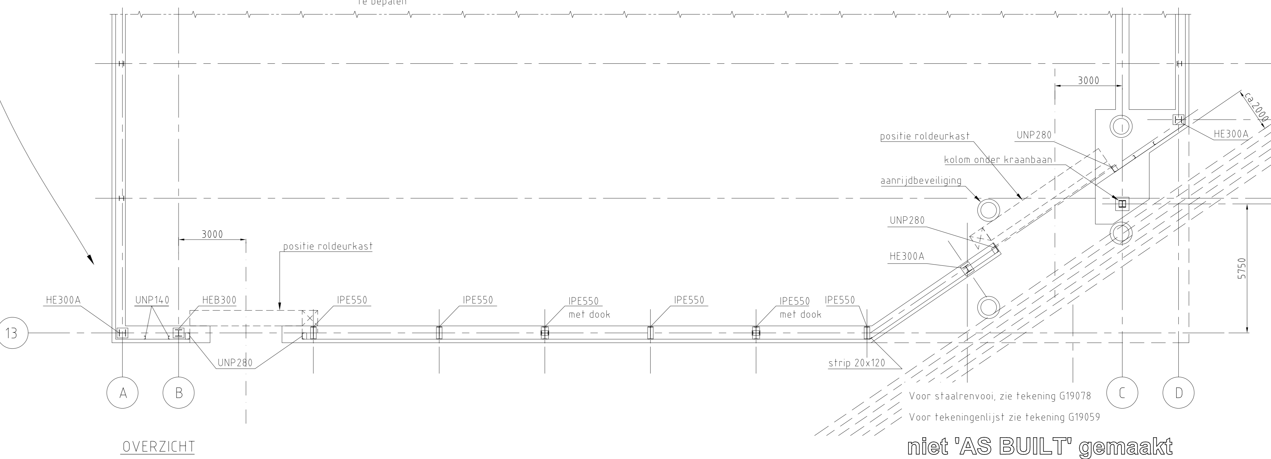
KOPGEVEL AS 13 (Z-W)
