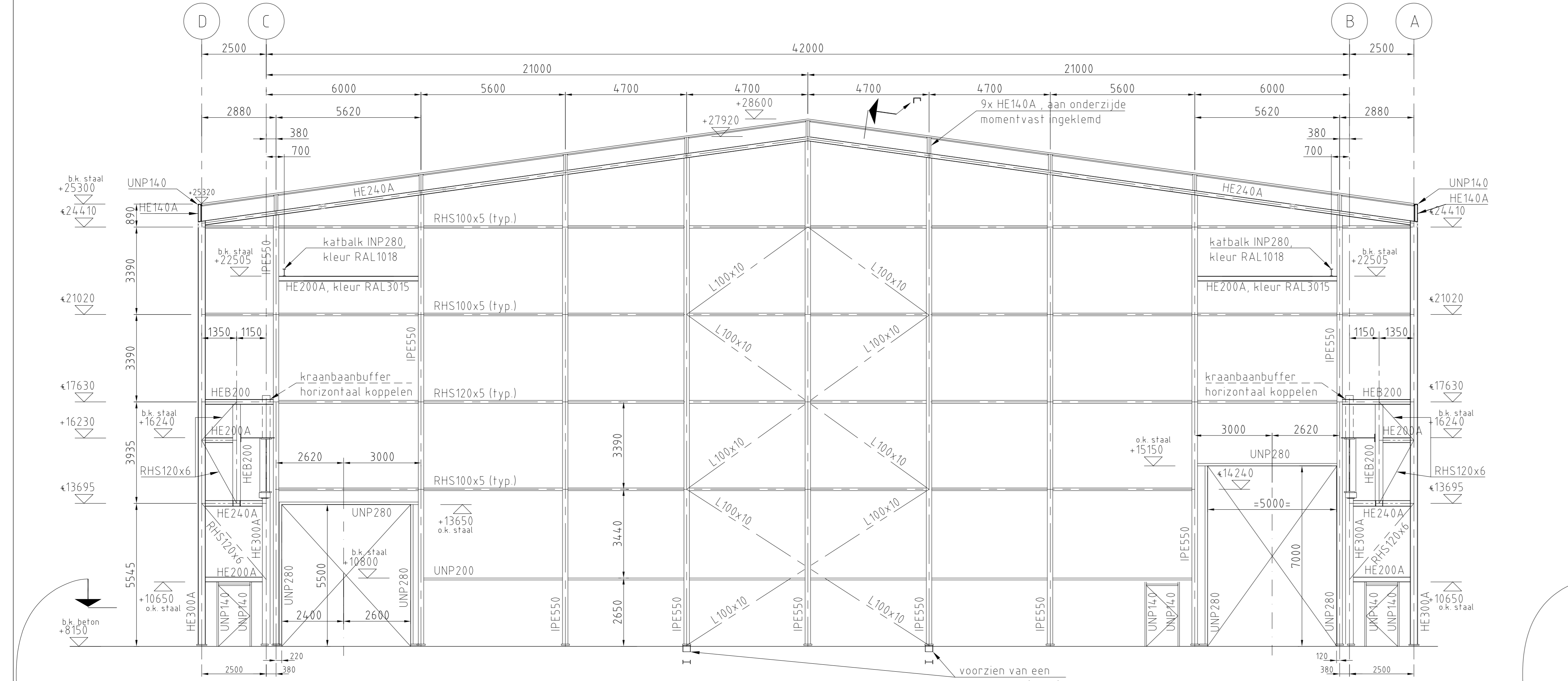
KOPGEVEL AS 1 (N-O)
