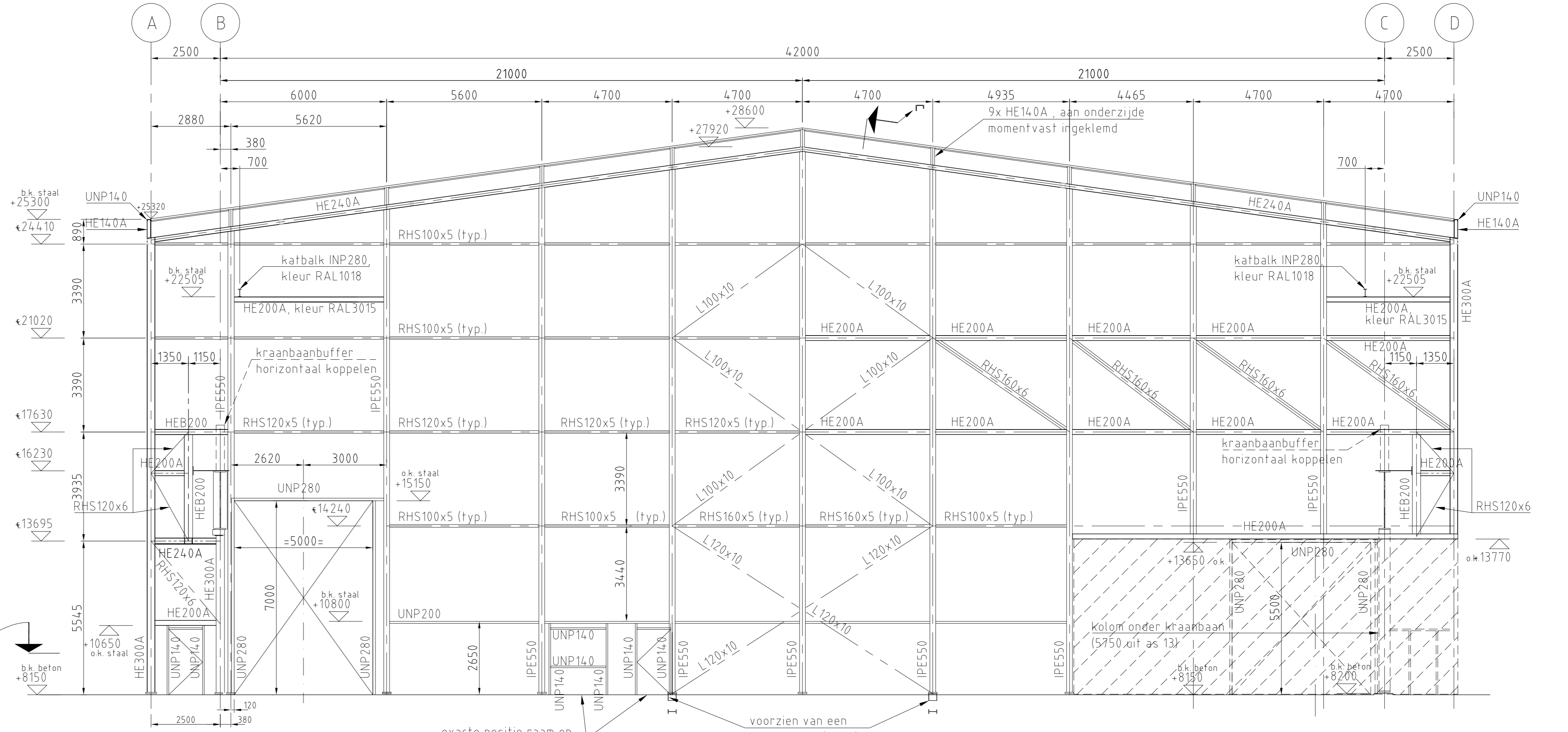
KOPGEVEL AS 13 (Z-W)
