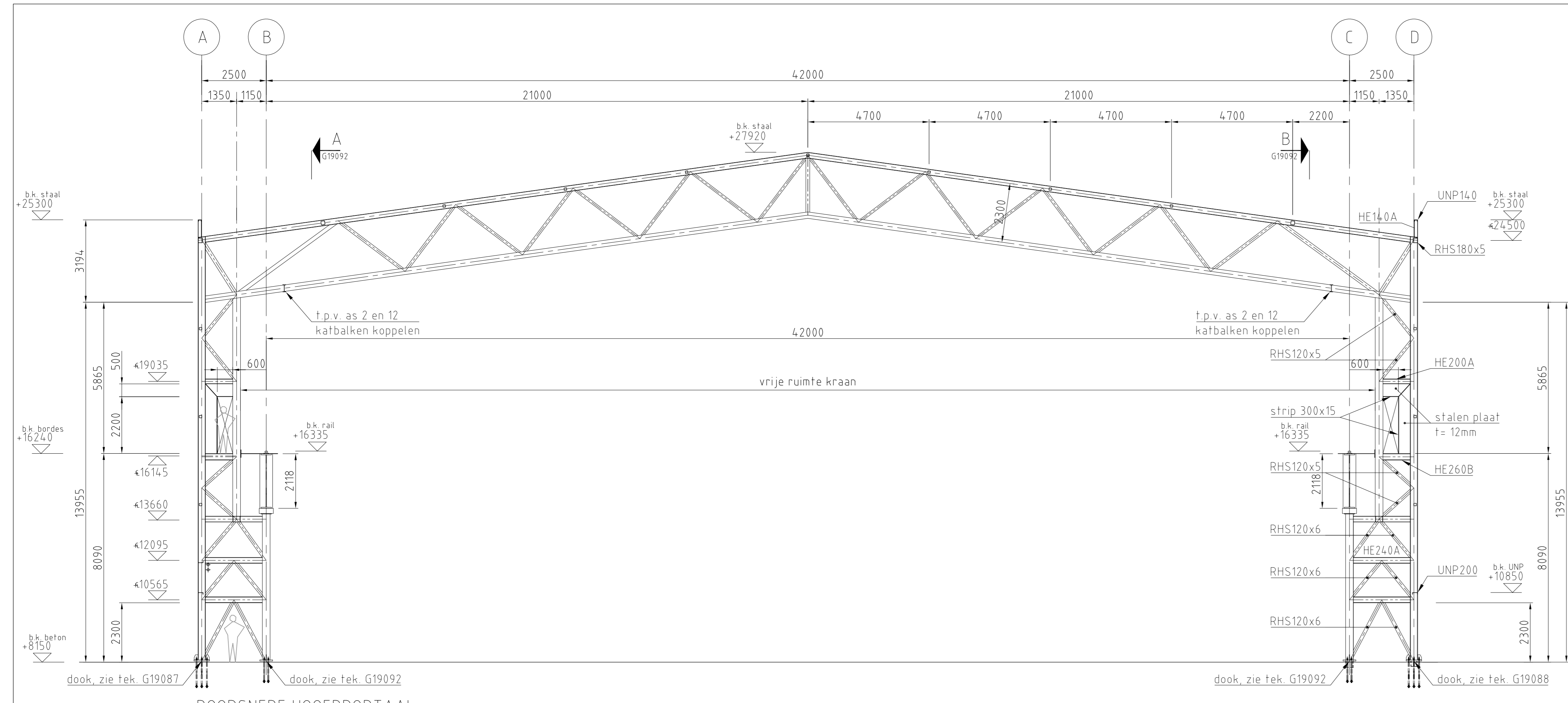
DOORSNEDE HOOFDPORTAAL
