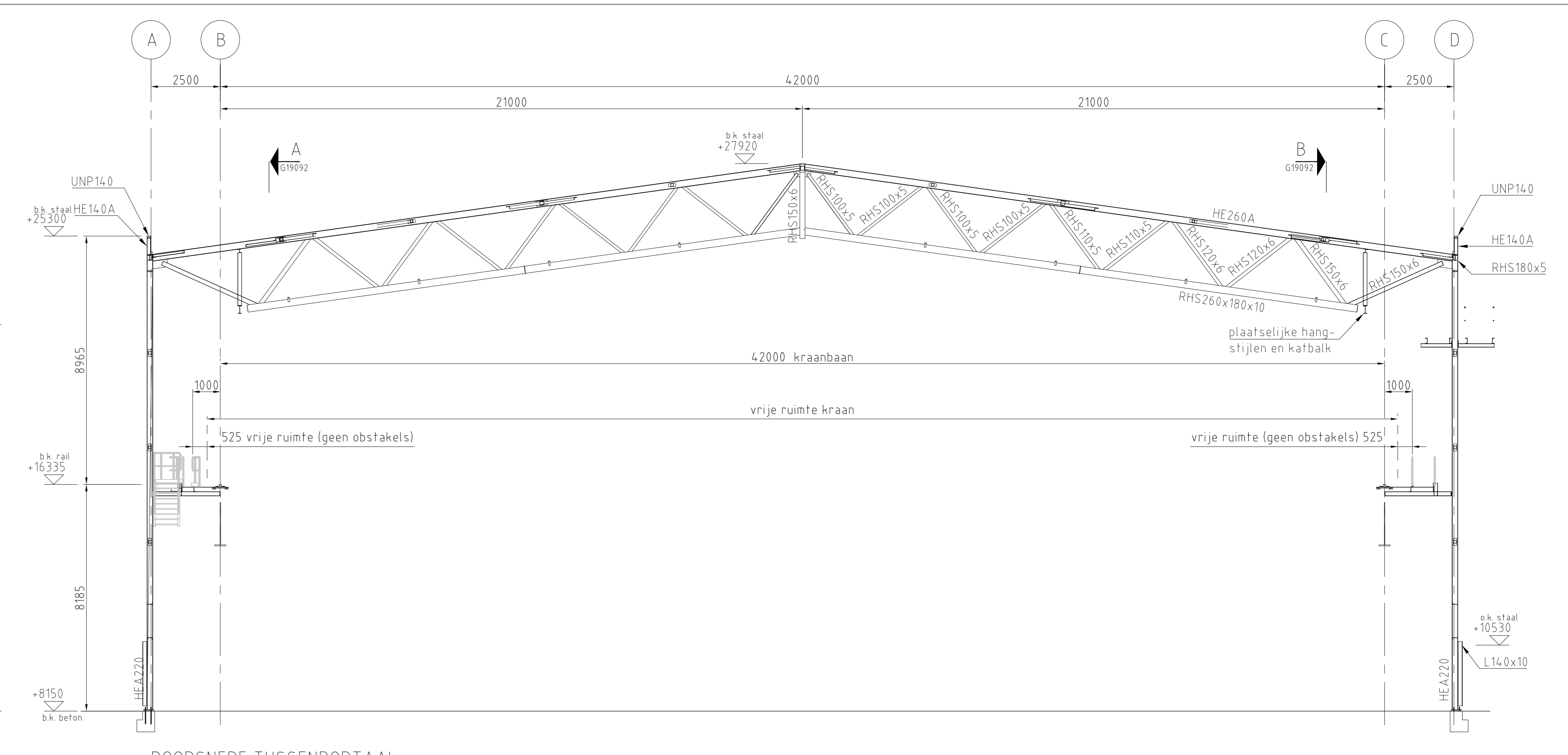
DOORSNEDE TUSSENPORTAAL
