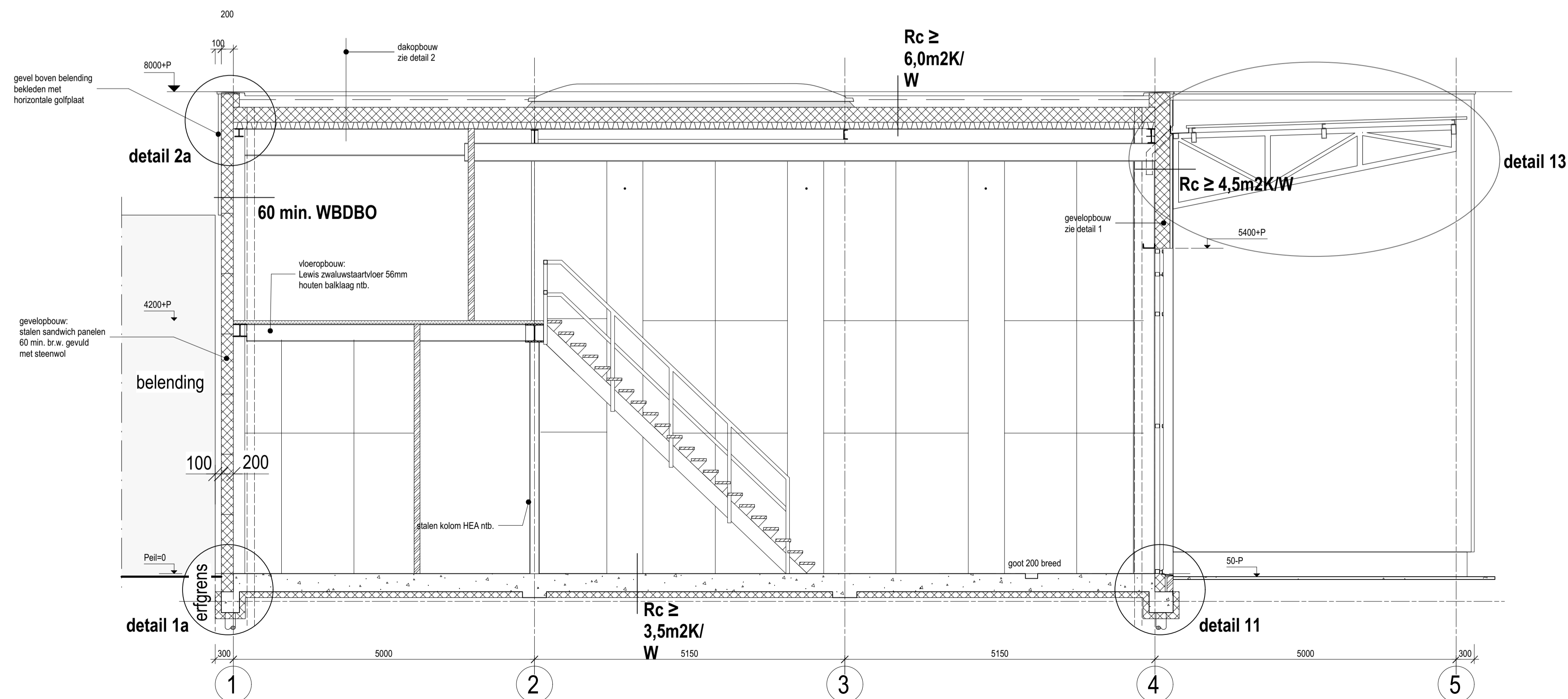
Doorsnede B-B
