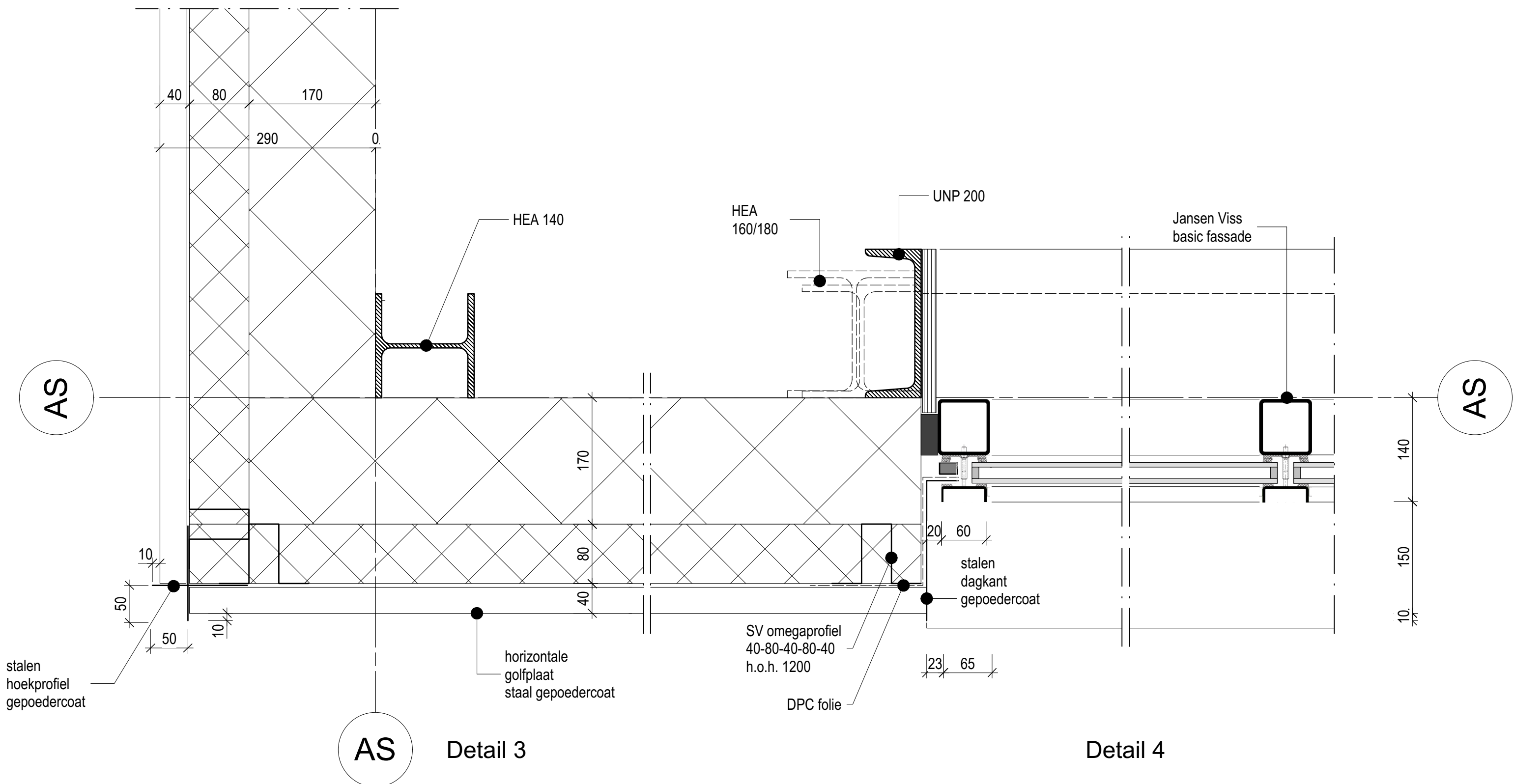
Detail 3 en 4 schaal 1 : 5 d.d. 15-11-2017
