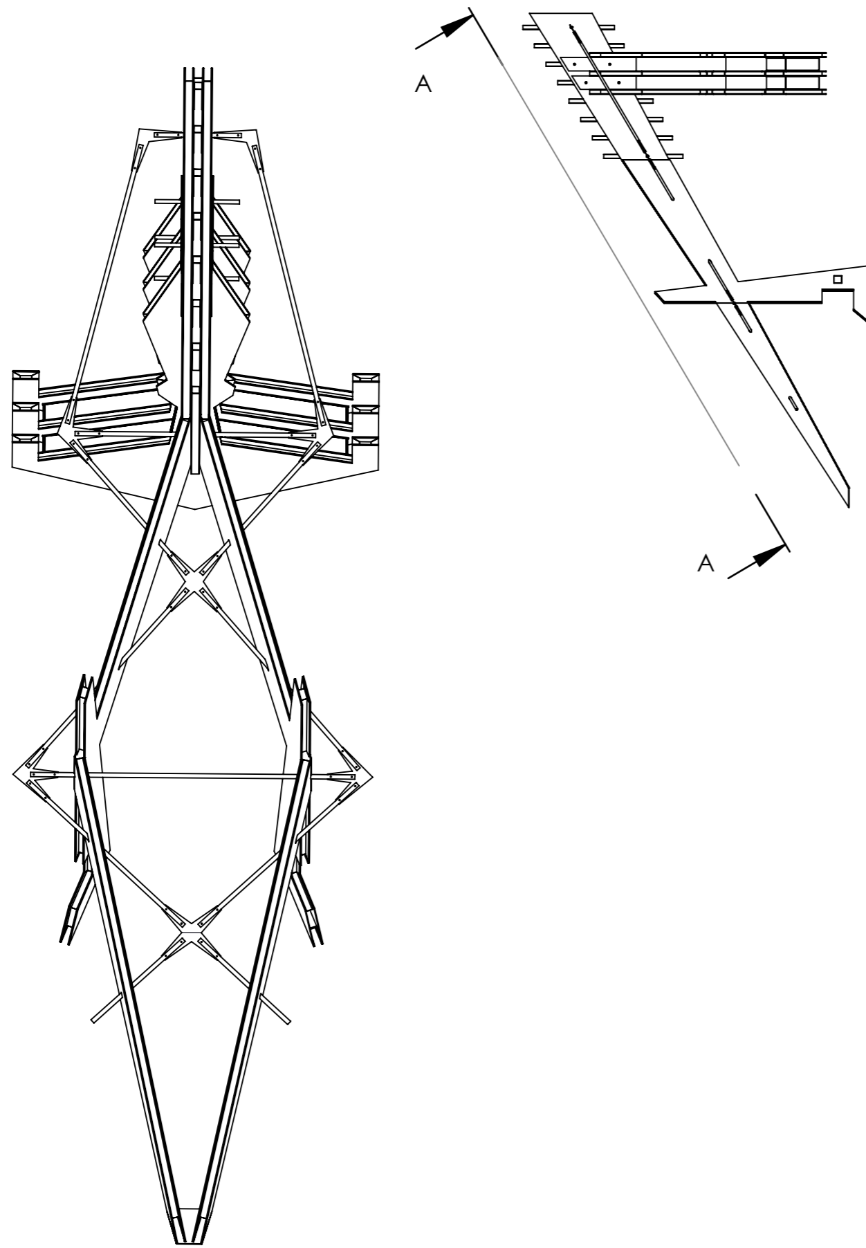
SECTION A-A aanzicht loodrecht op koppelplaten SCALE 1 : 50
