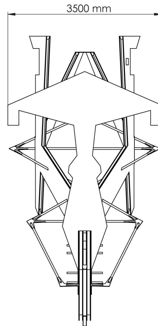
boven-aanzicht
