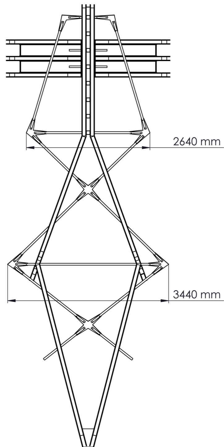
Voor-aanzicht
