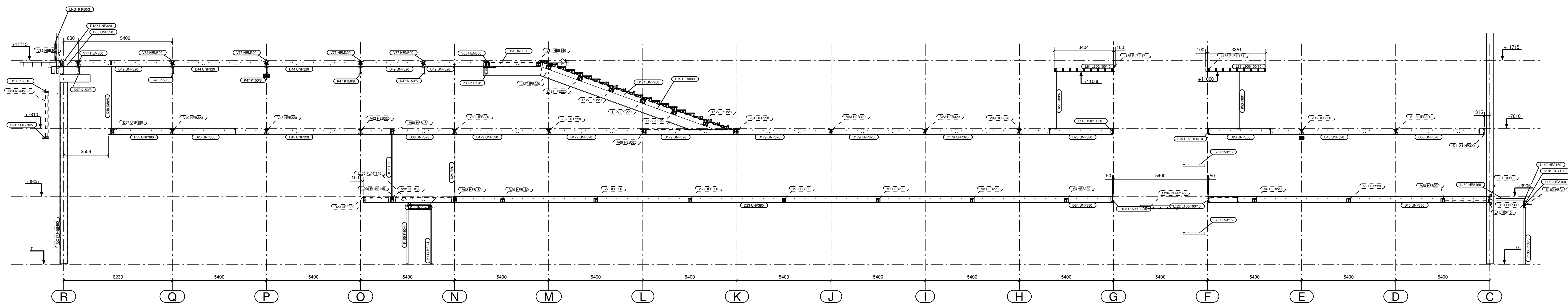
DOORSNEDE : AS-22/23
