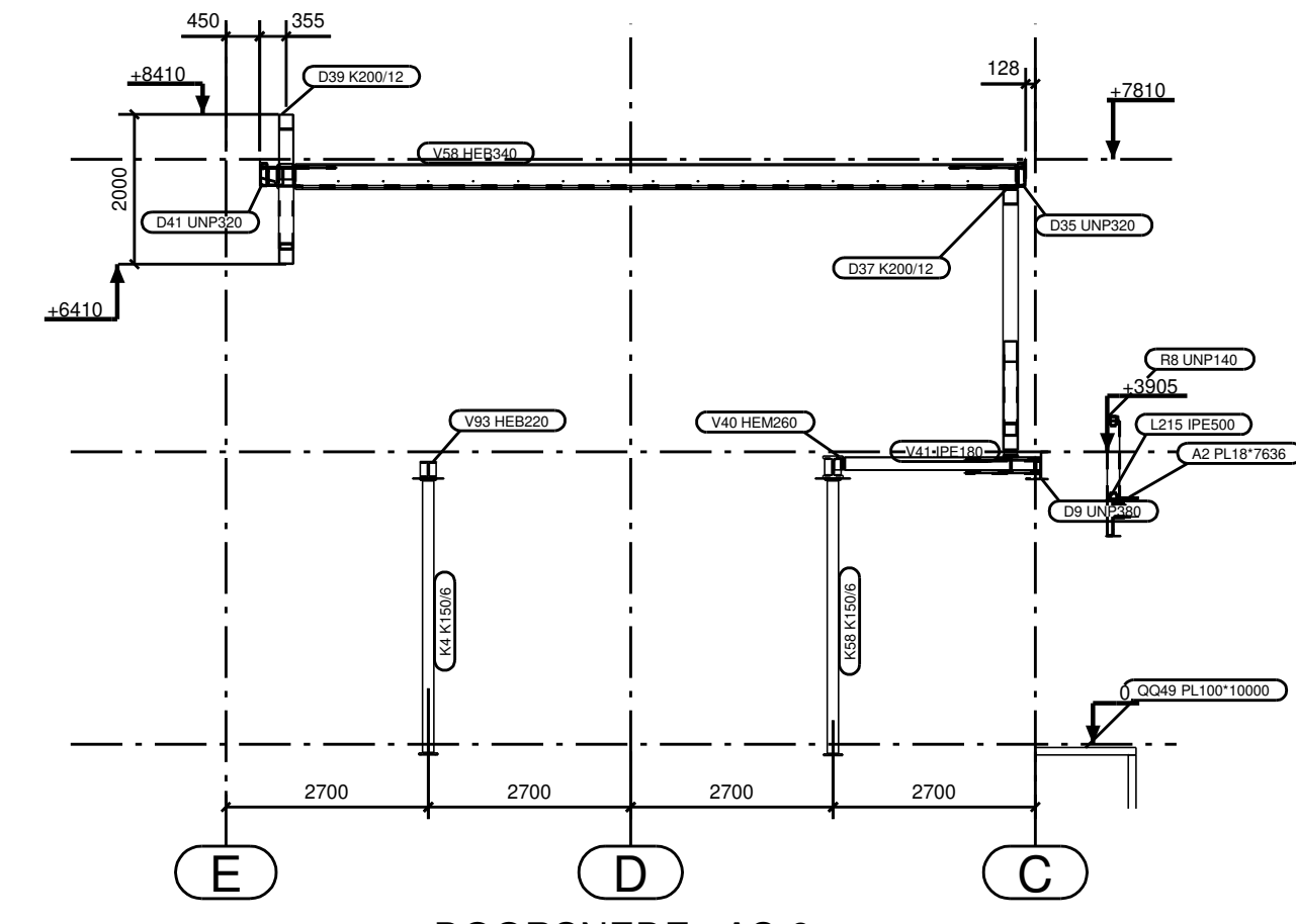
DOORSNEDE : AS-9
