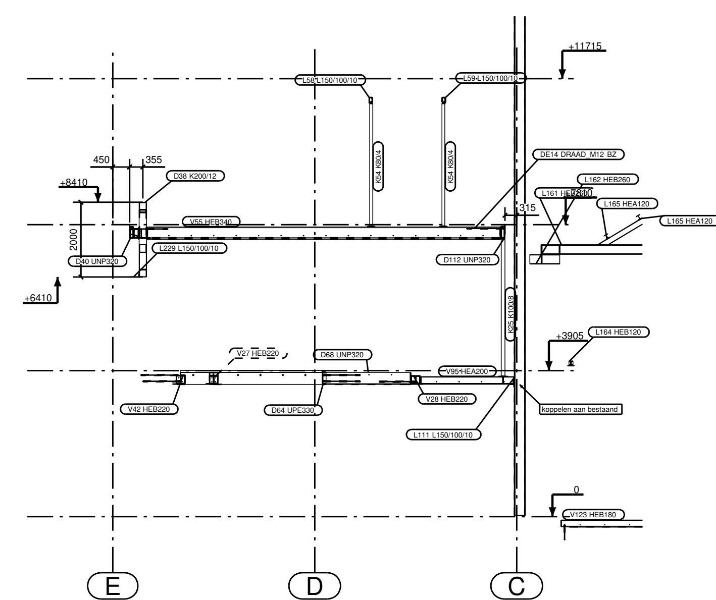
DOORSNEDE : AS-17
