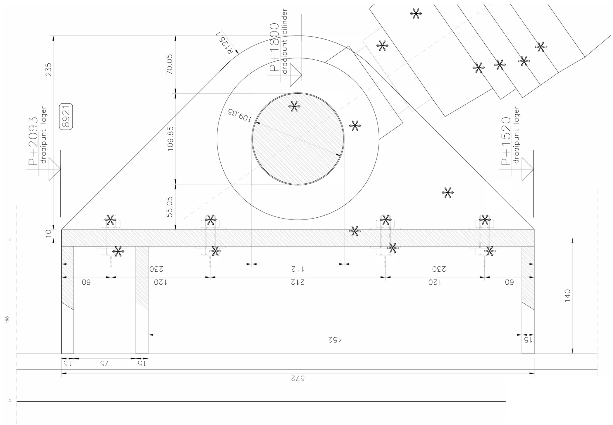
Bevestiging boomcilinder aan vloer
