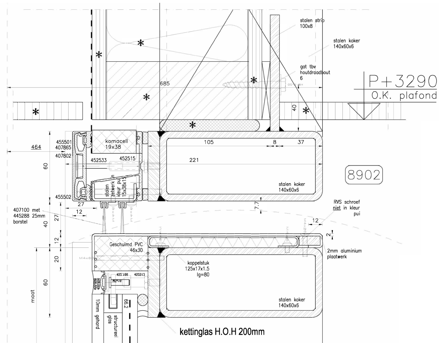
Detail bovenaansluiting hefdeur
