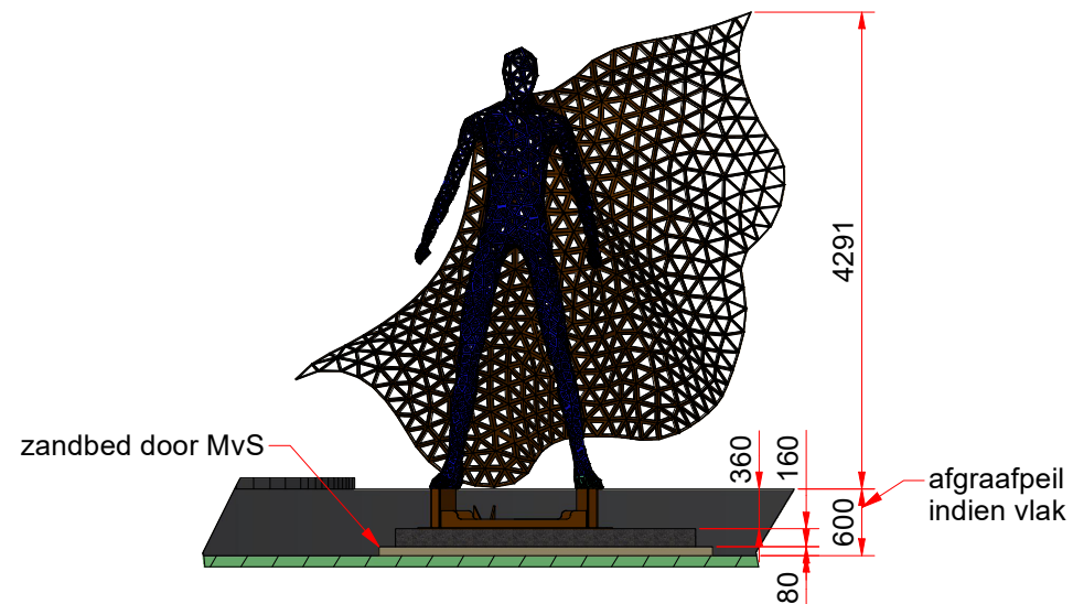
A-A (1 : 75)
