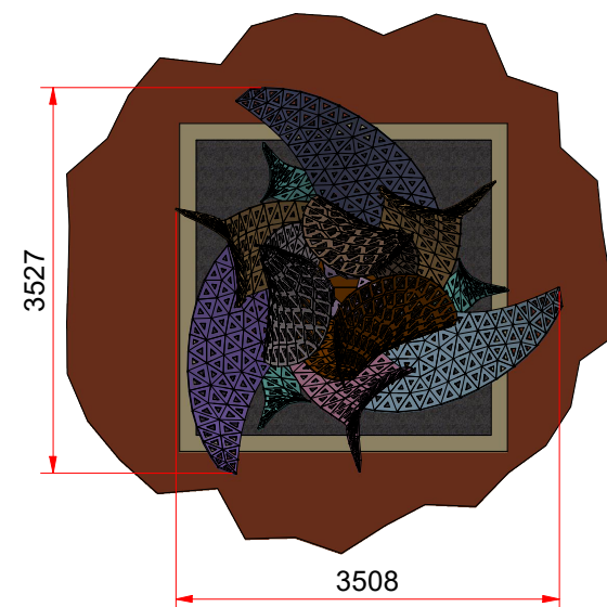
B ( 1 : 75 )
