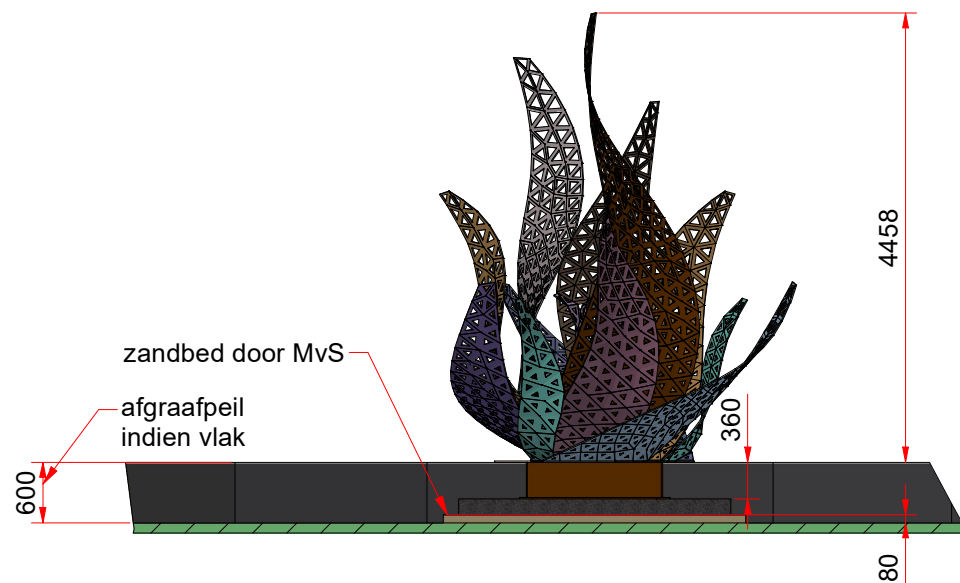
A-A ( 1 : 75 )
