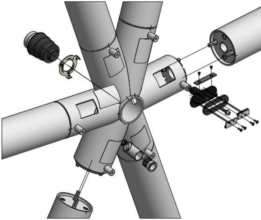
ISOMETRIE (GE-EXPLODEERD)
