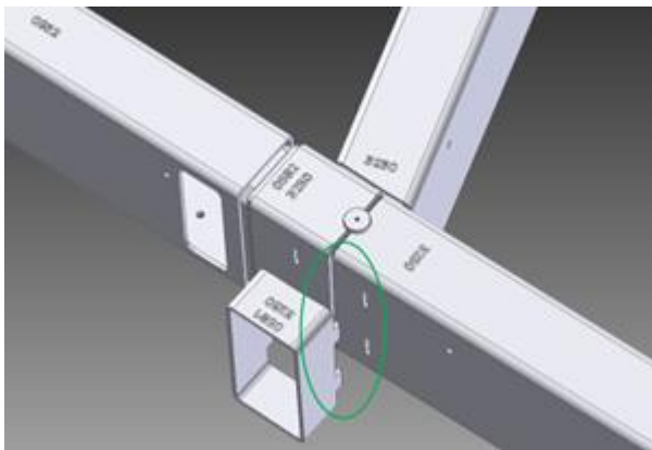
Detail combinatieknoop gelast en gebout
