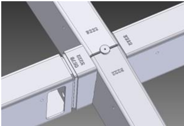
Detail combinatieknoop
