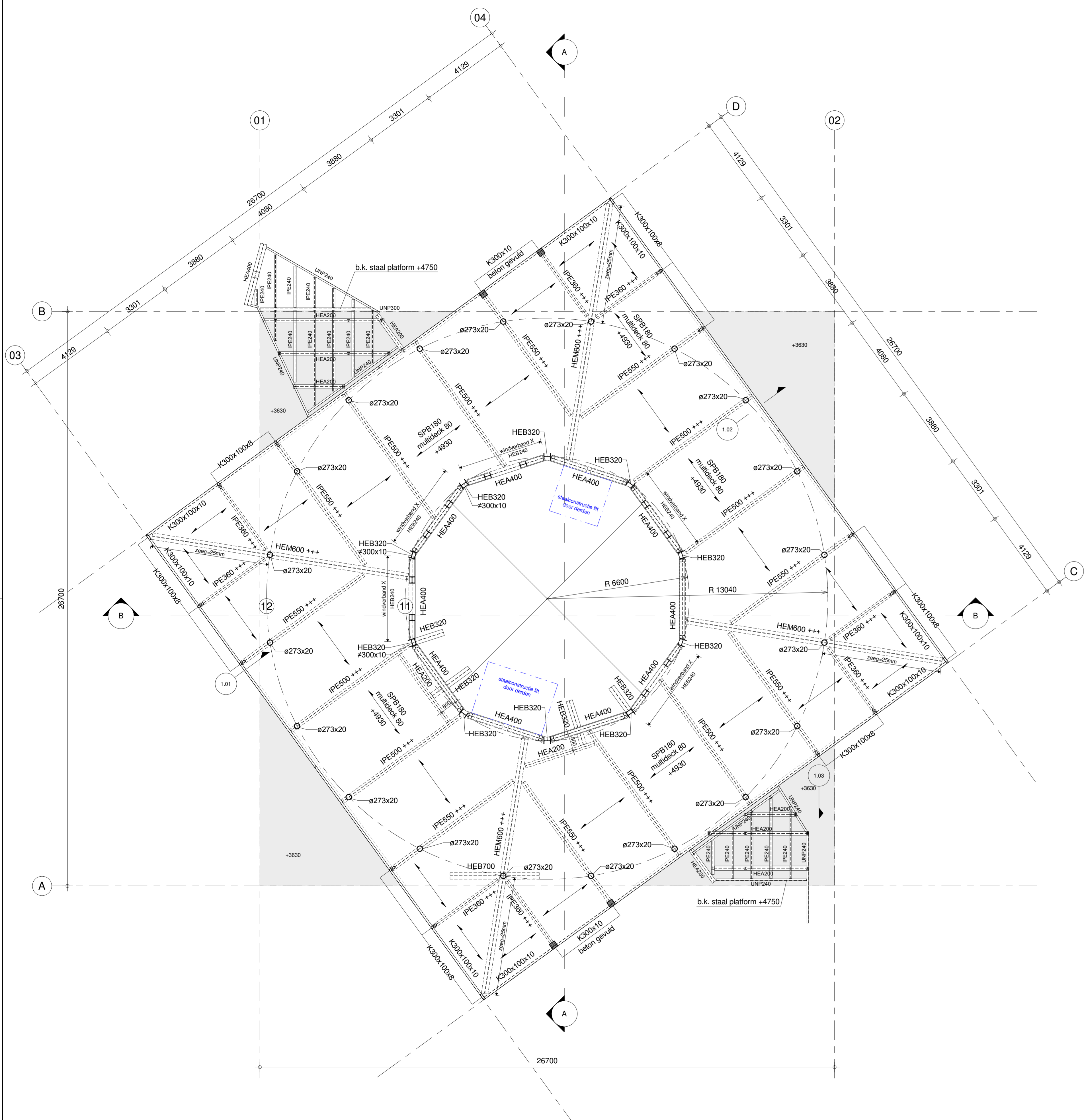
Eerste Verdiepingsvloer
