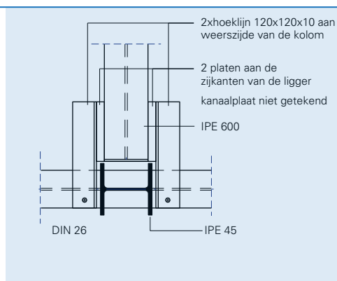
Oplegdetail ligger bij de tuinbouwkas op het Gorlaeus-staal aan weerszijden (horizontale doorsnede).
