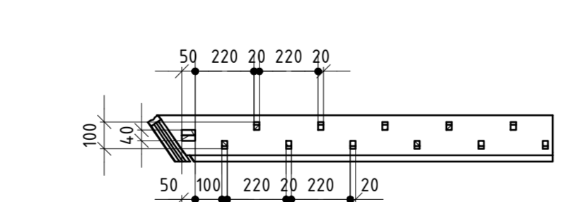
Doorsnede J-J SCHAAL 1 : 20
