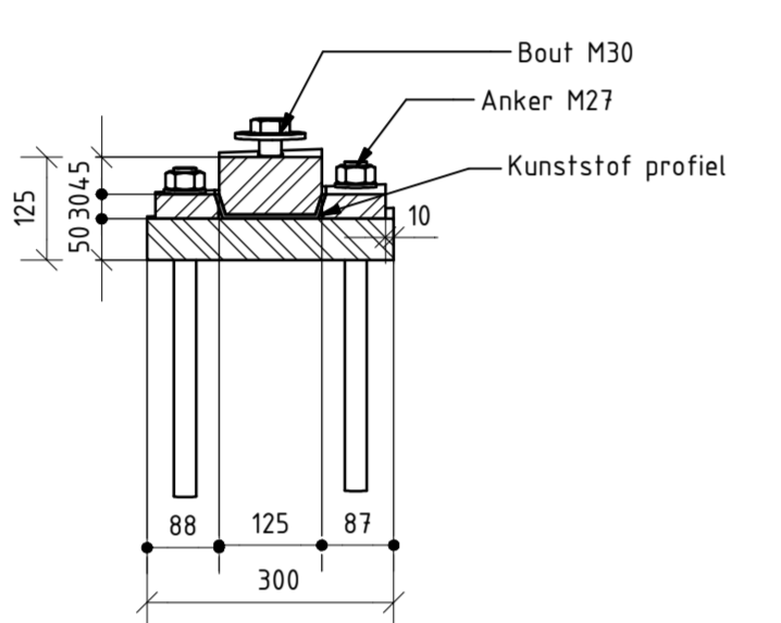
Doorsnede G-G SCHAAL 1 : 10
