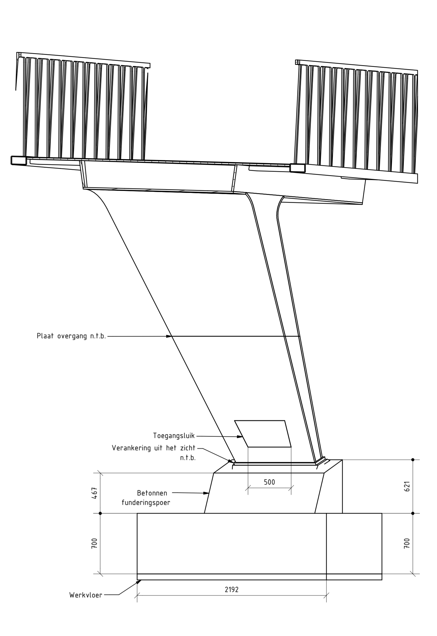
Doorsnede P-P SCHAAL 1 : 25
