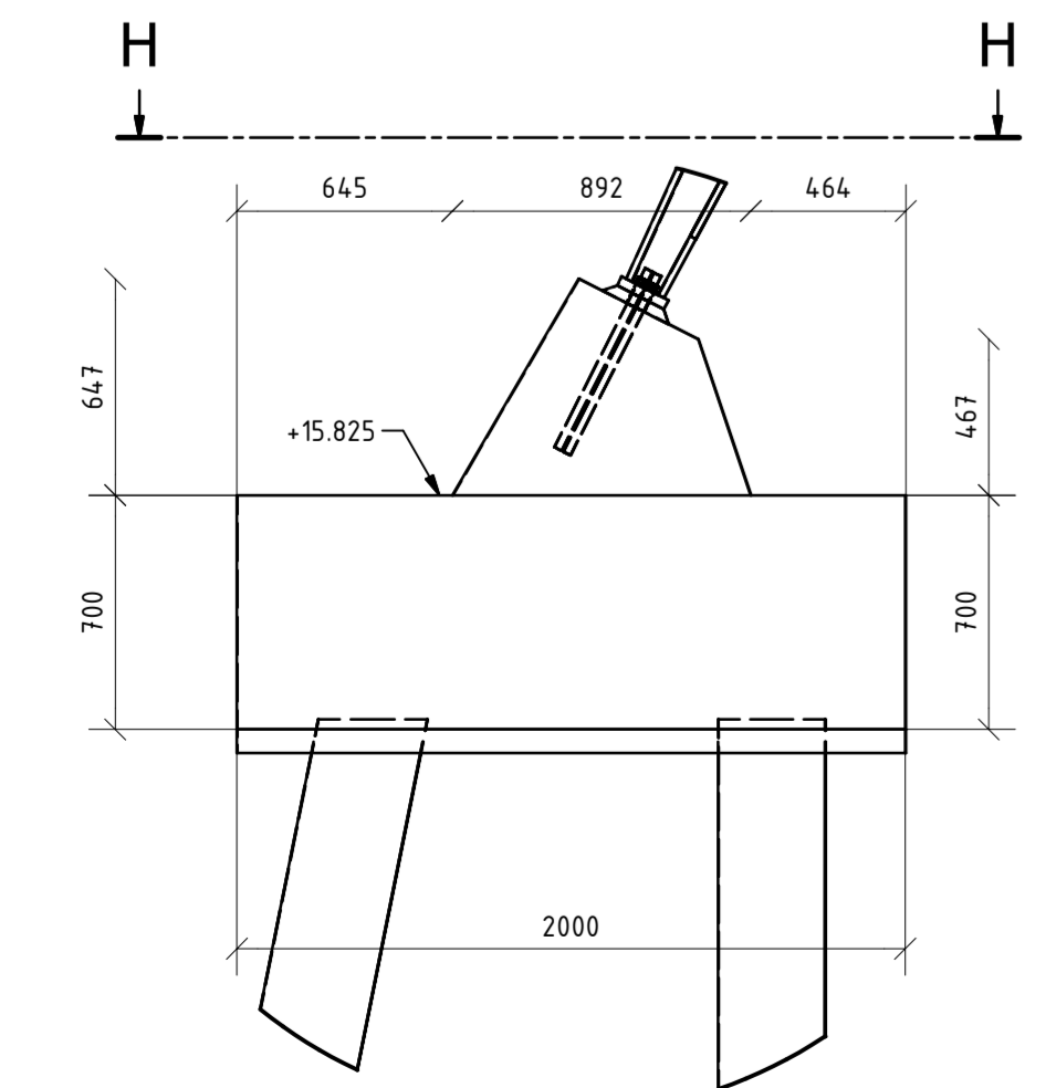
Detail 2 SCHAAL 1 : 25
