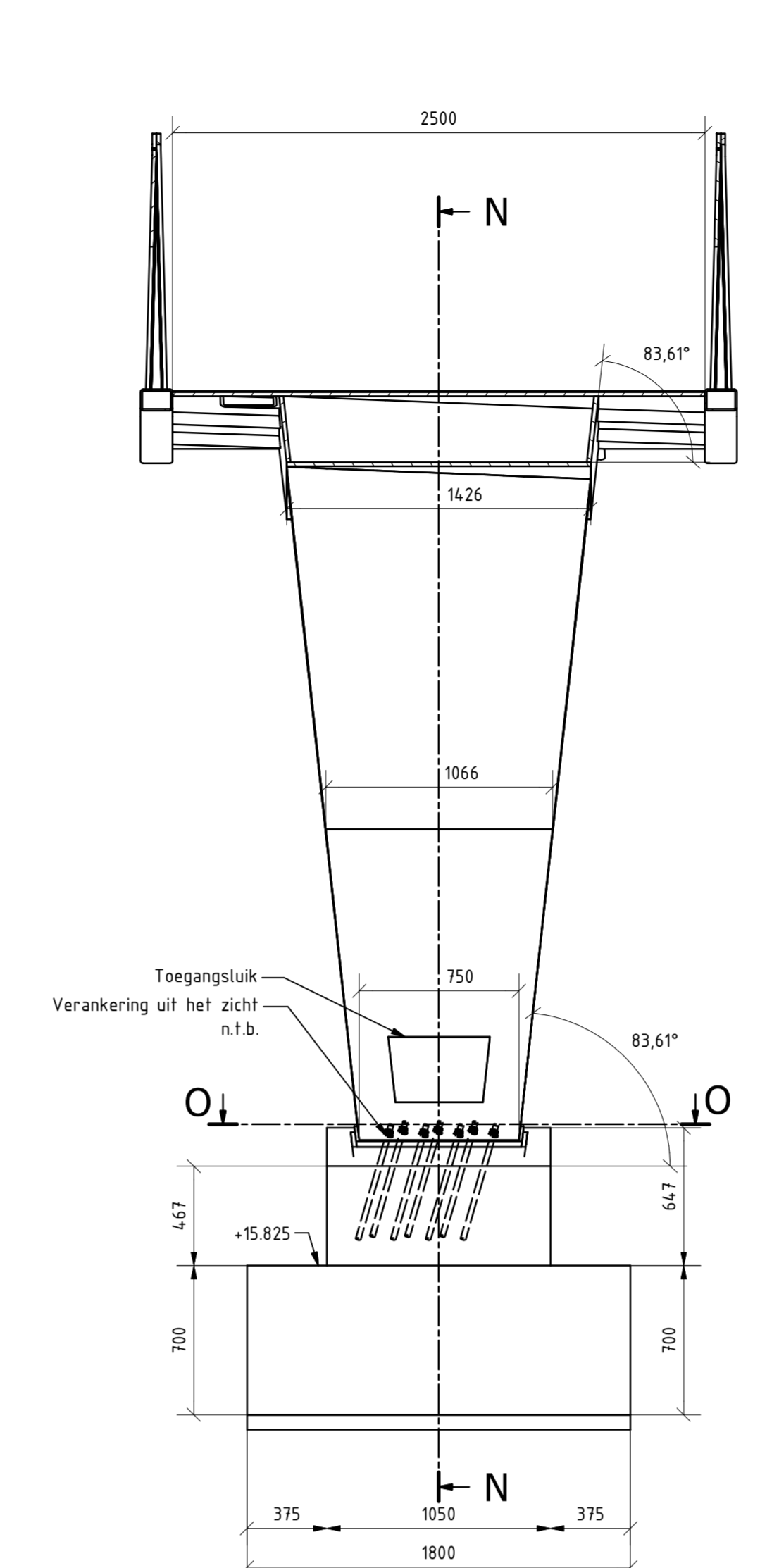
Doorsnede M-M SCHAAL 1 : 25
