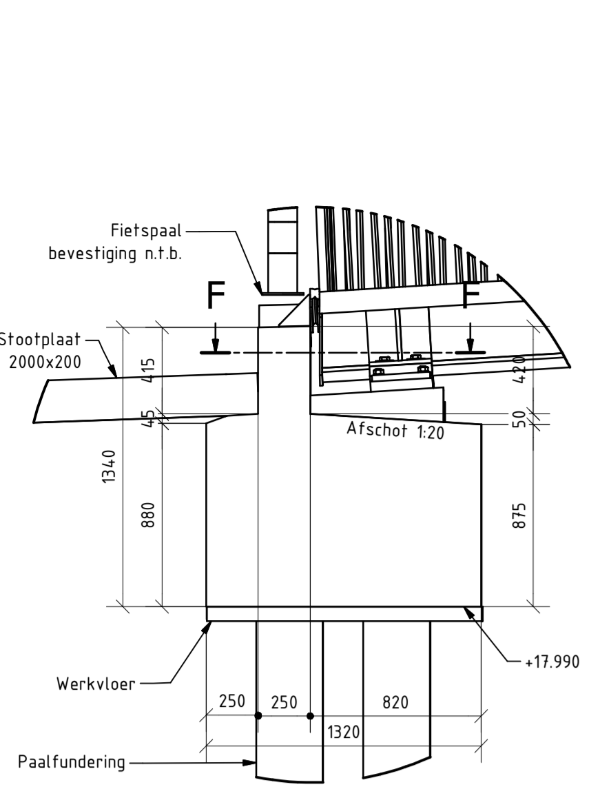
Detail 1 SCHAAL 1 : 25 Zijaanzicht landhoofd
