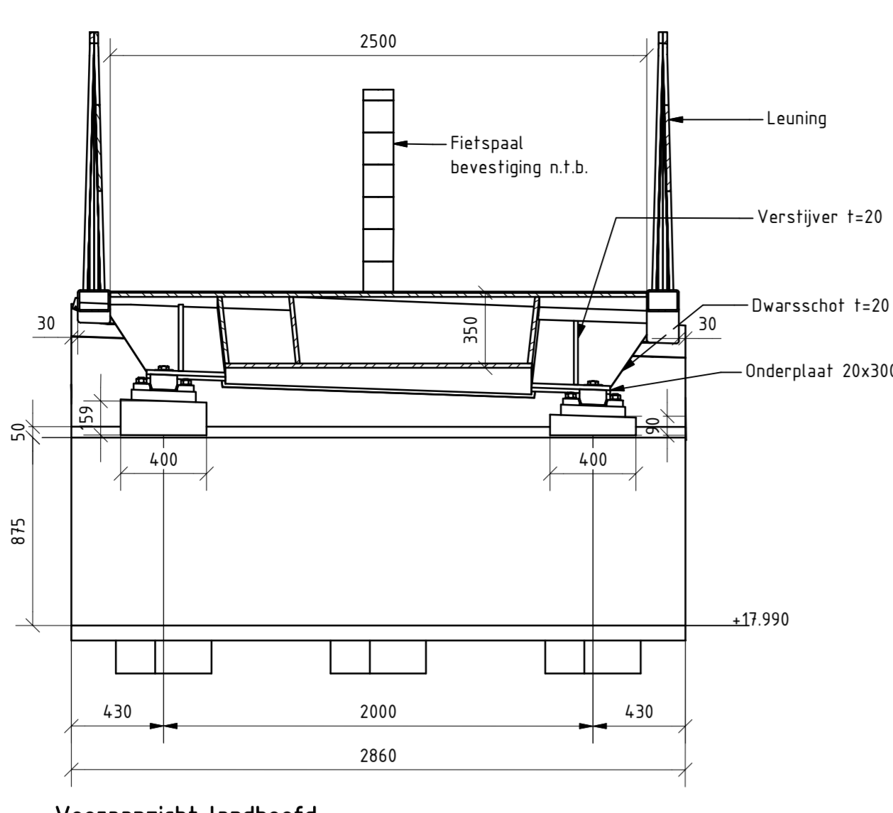
Vooraanzicht landhoofd SCHAAL 1 : 25
