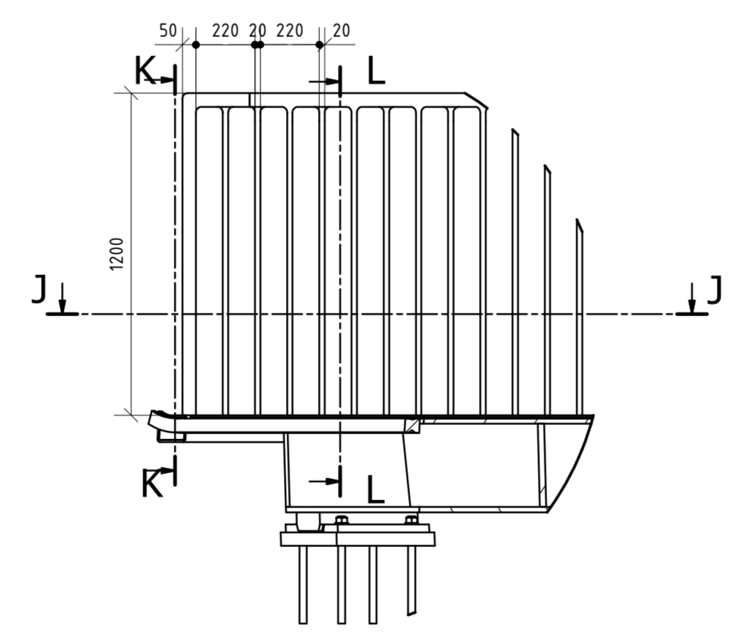
Detail 3 SCHAAL 1 : 20 Leuning
