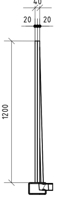
Doorsnede K-K SCHAAL 1 : 20
