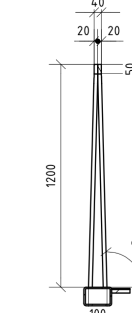
Doorsnede L-L SCHAAL 1 : 20
