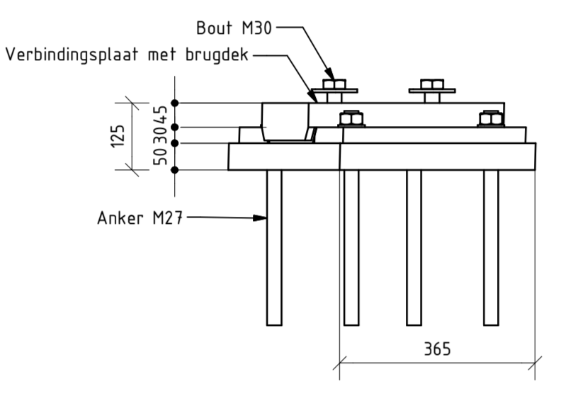
Vooraanzicht oplegging SCHAAL 1 : 10
