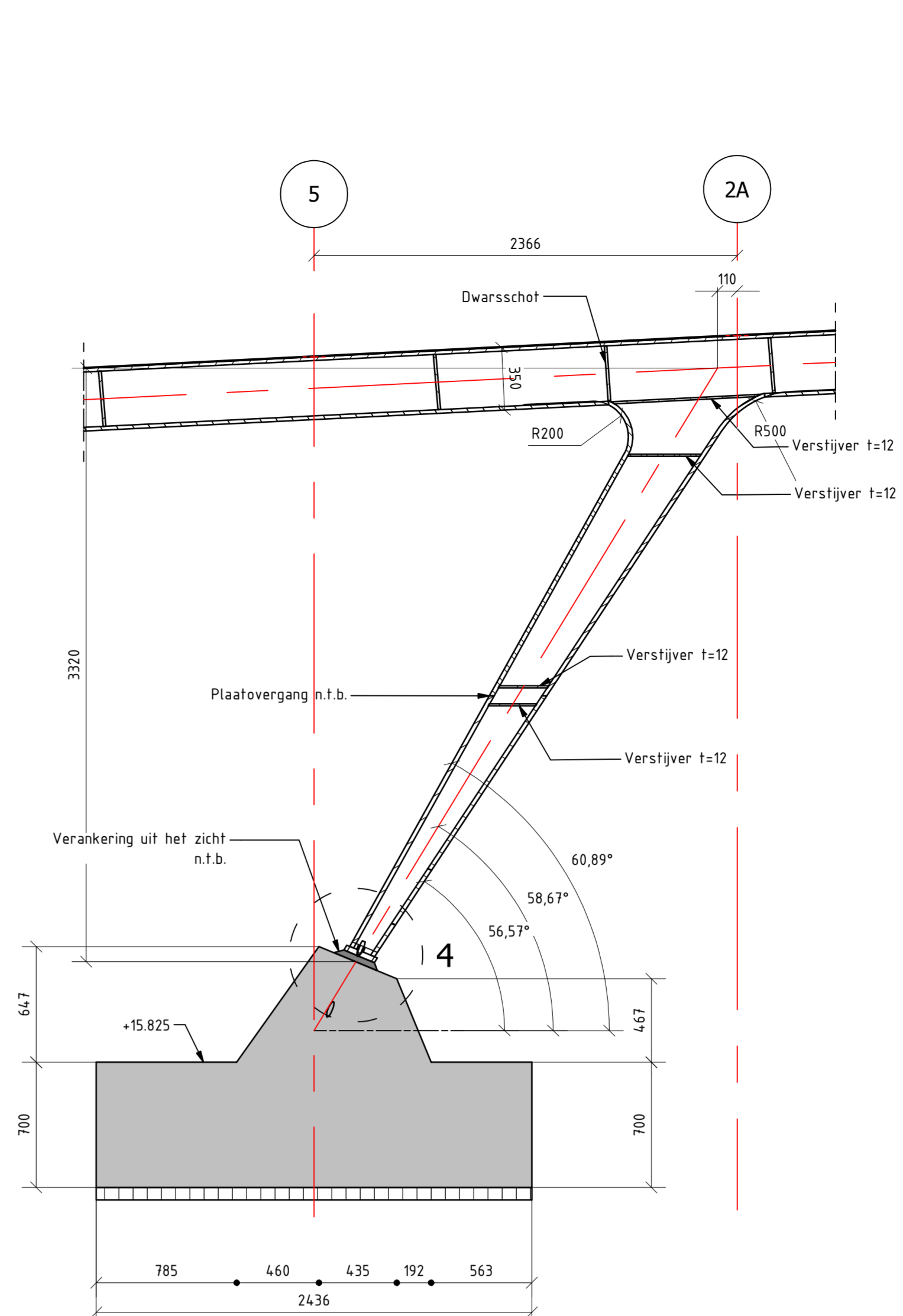
Doorsnede N-N SCHAAL 1 : 25
