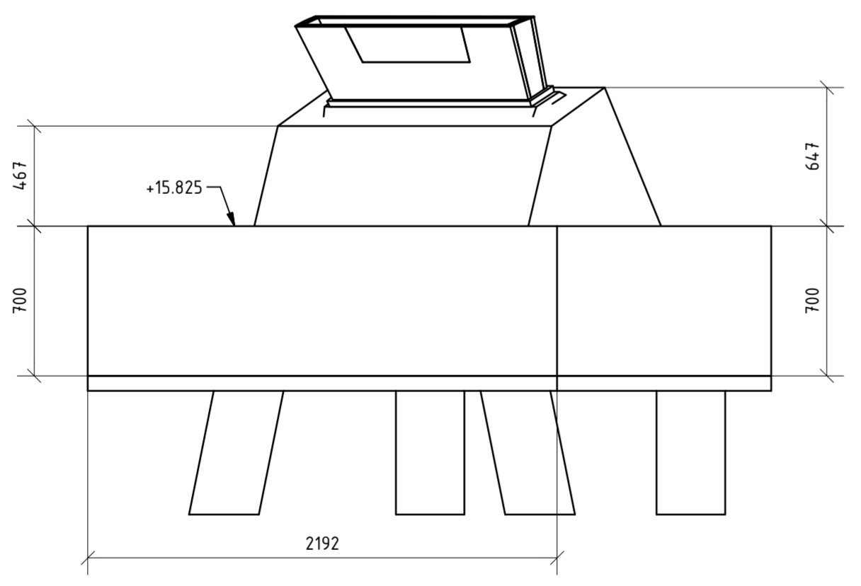
Aanzicht AC SCHAAL 1 : 25
