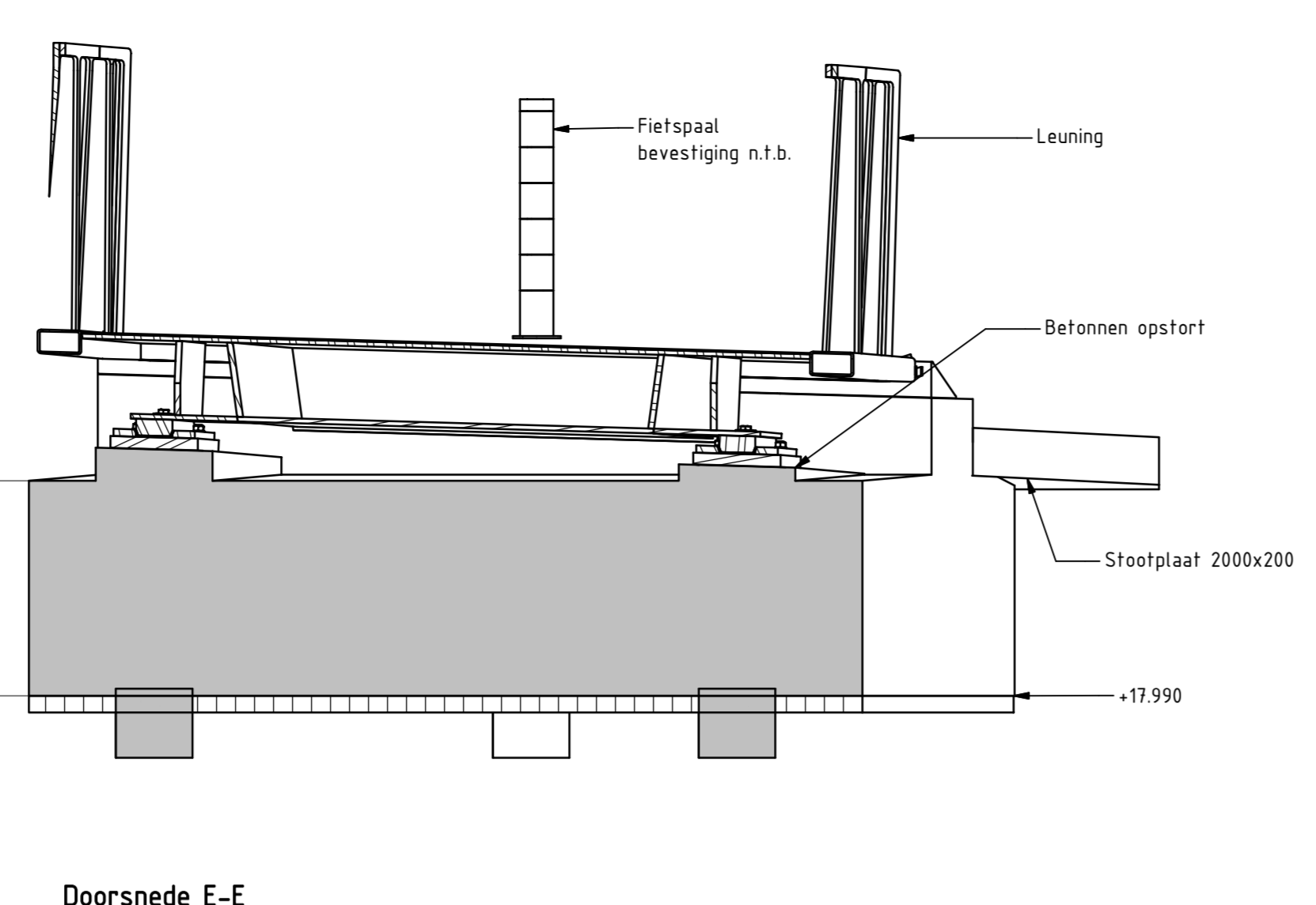
Doorsnede E-E SCHAAL 1 : 25
