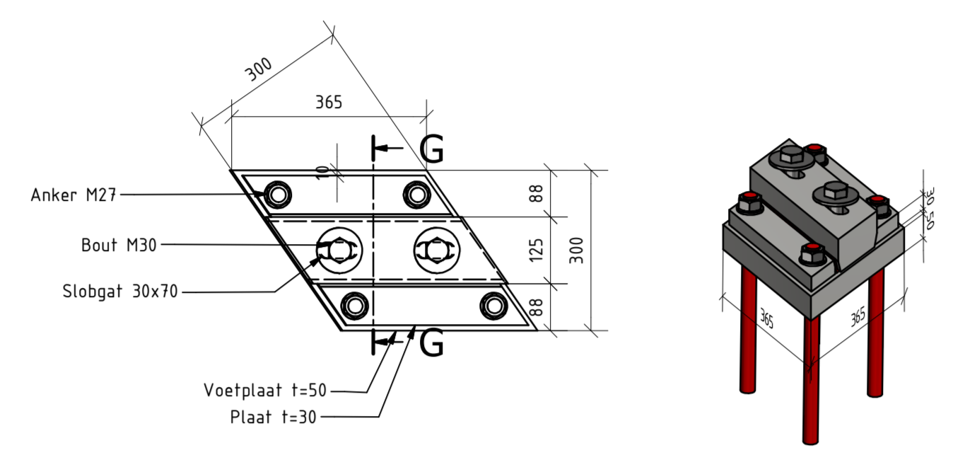
Oplegging bovenaanzicht SCHAAL 1 : 10
