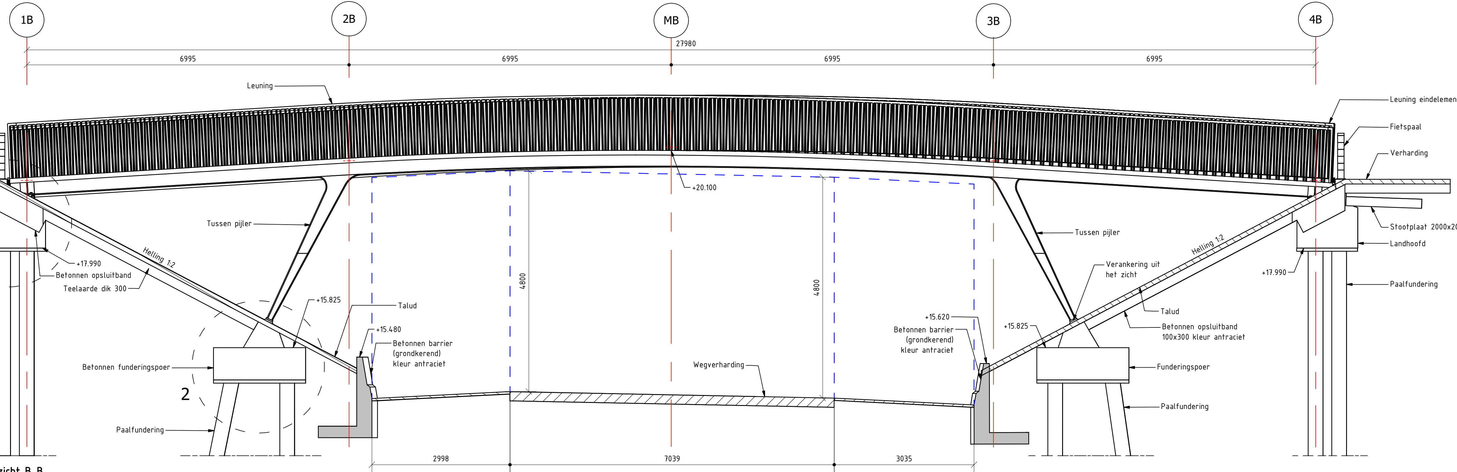
Aanzicht B-B SCHAAL 1 : 50 Zijaanzicht
