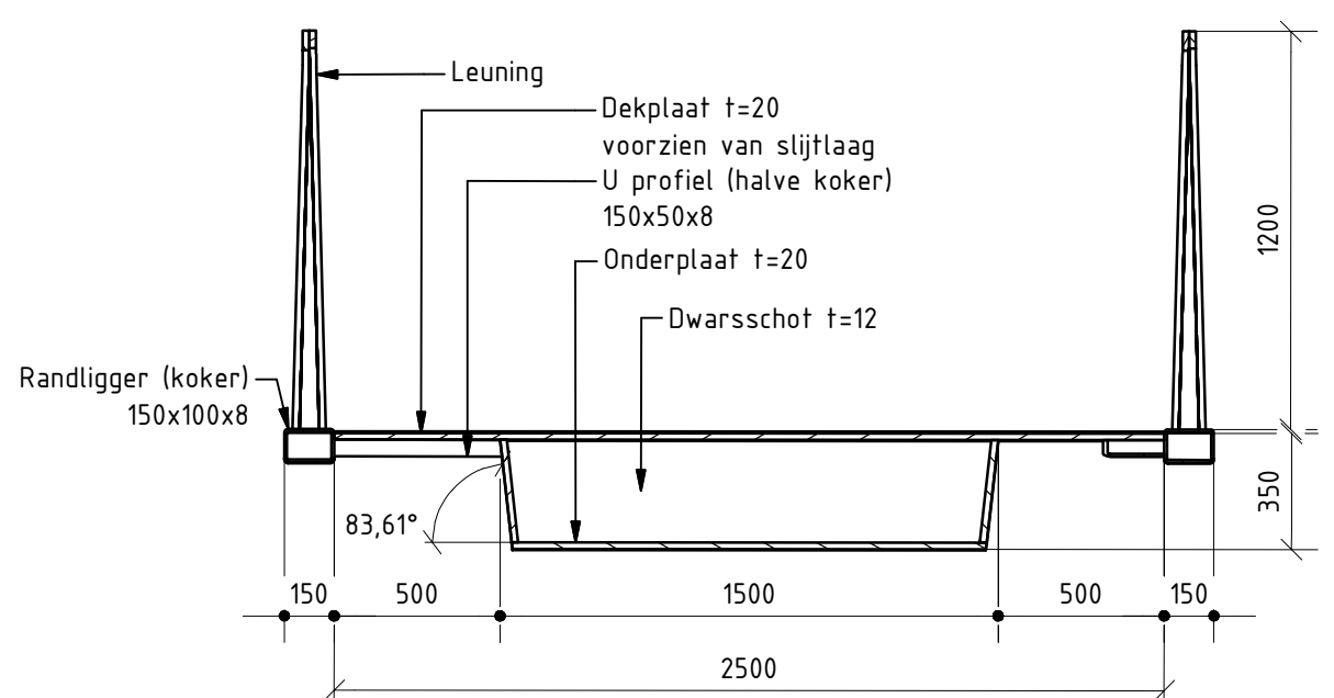
Doorsnede D-D SCHAAL 1 : 25 Dwaarsdoorsnede brugdek
