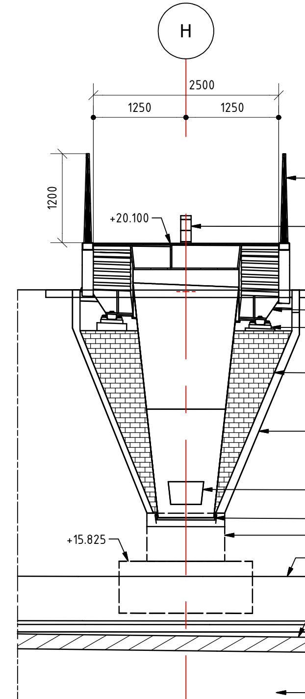
Doorsnede C-C SCHAAL 1 : 50 Dwaarsdoorsnede
