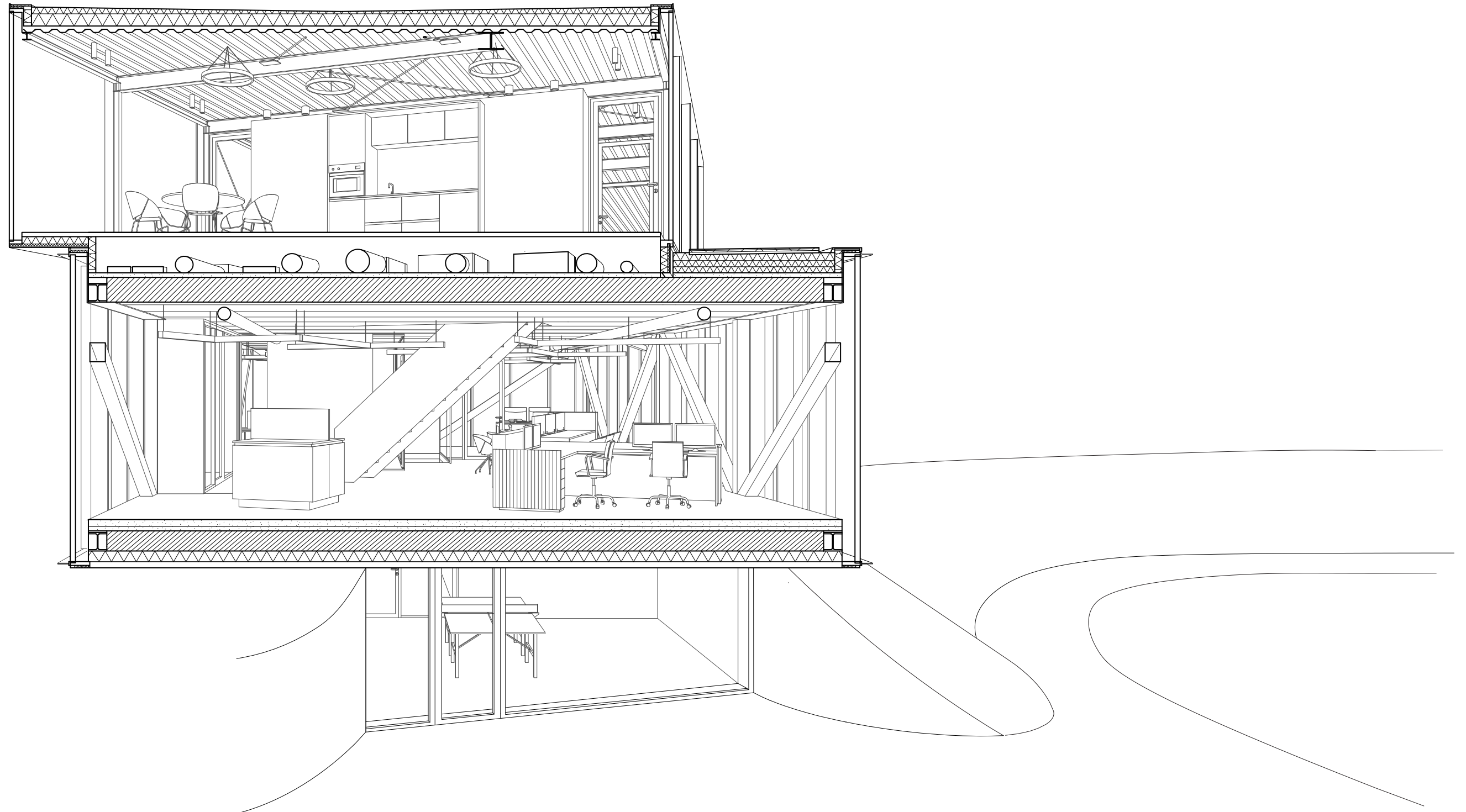
doorsnede 1:50
