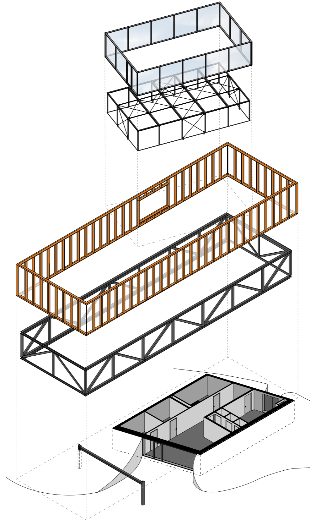
Axonometrie
