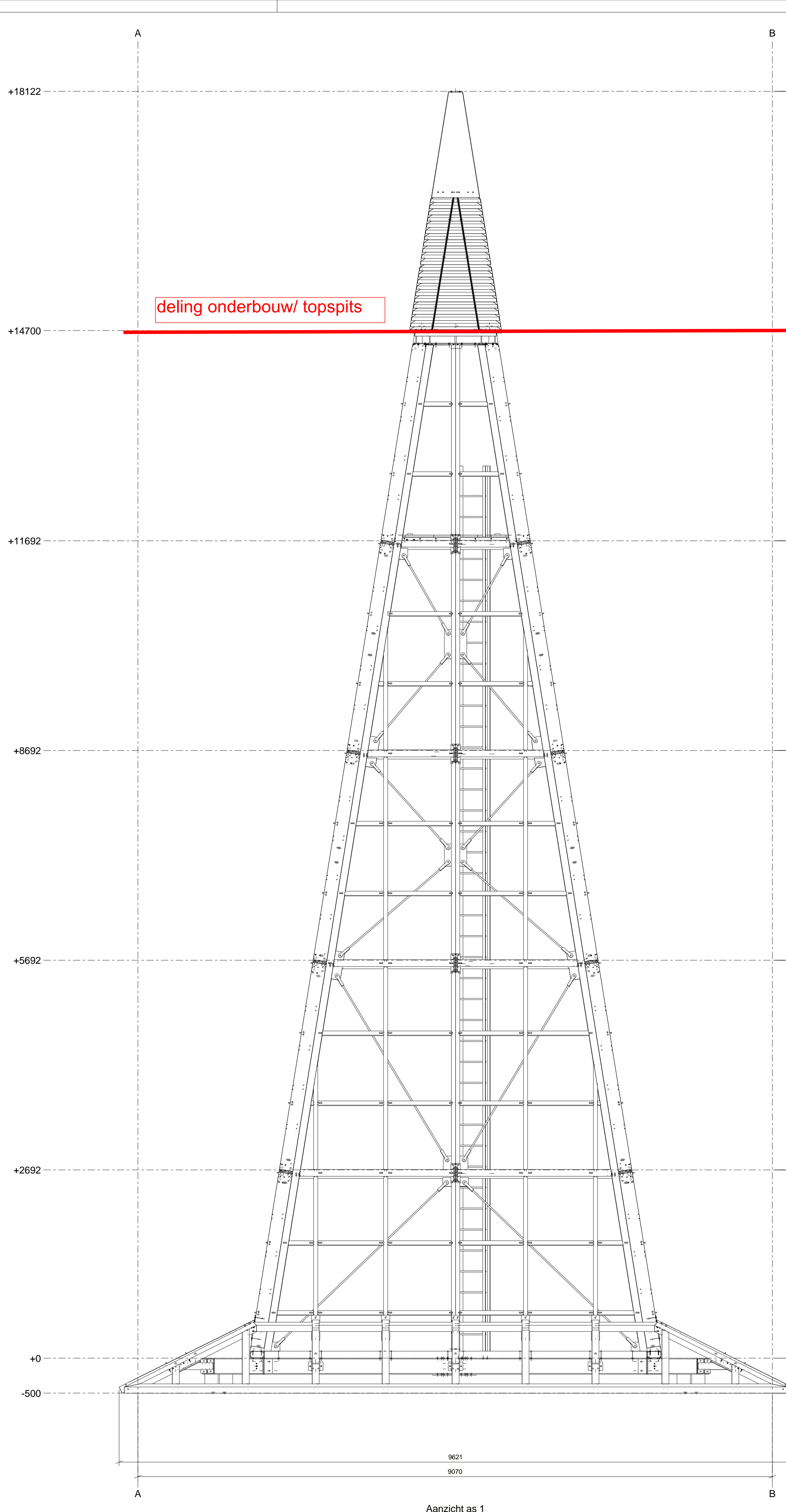
Aanzicht as 1 1:35
