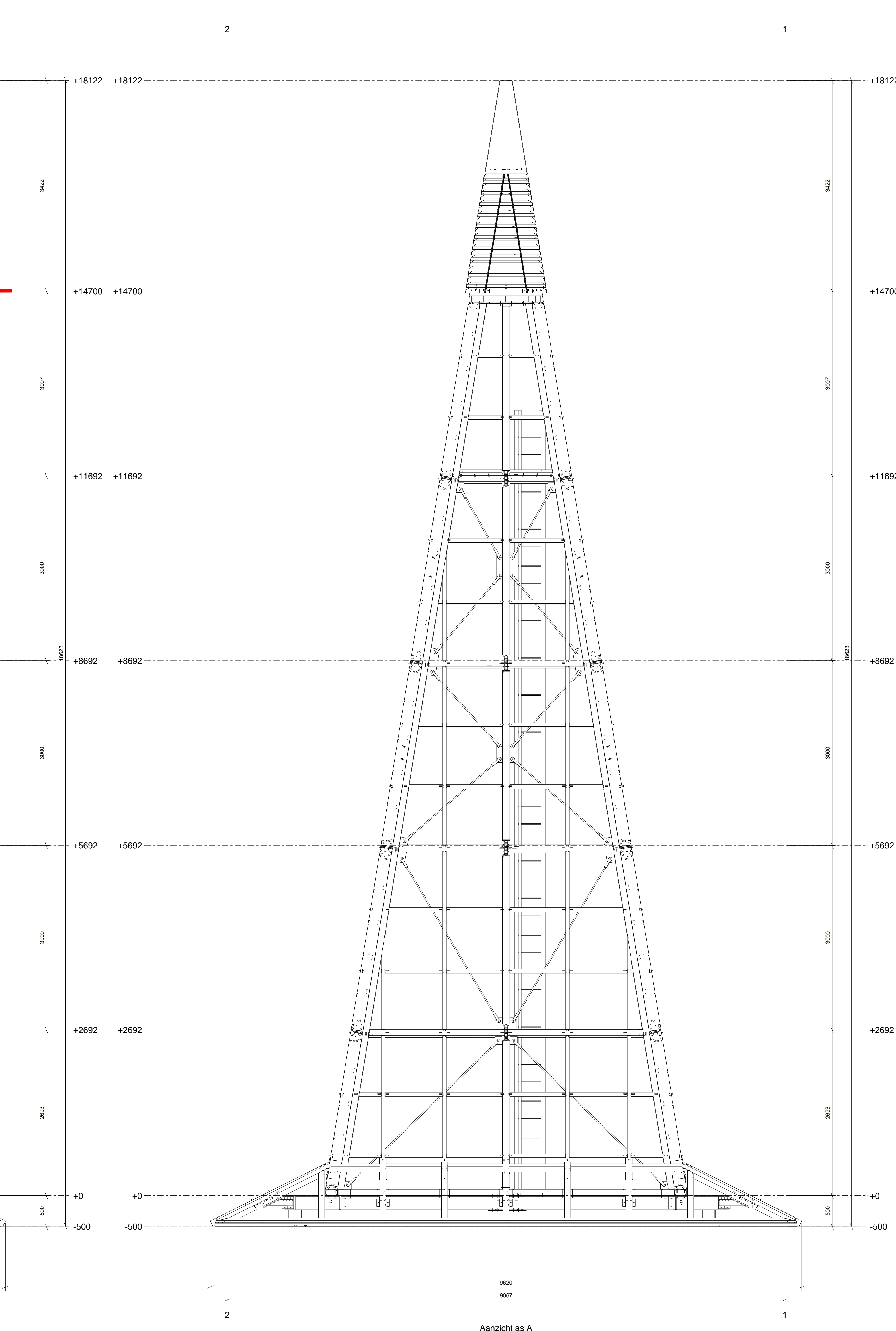
Aanzicht as A 1:35
